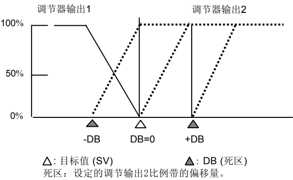
①2-输出加热/冷却动作输出特性
