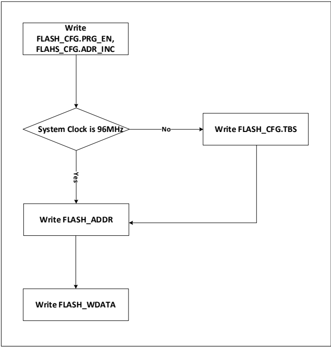
图 6-5 FLASH 模块编程操作流程
