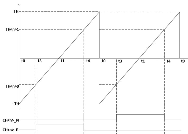
图 12-8 MCPWM 时序 TH&lt;n&gt;0 和 TH&lt;n&gt;1-中心对齐推挽模式
