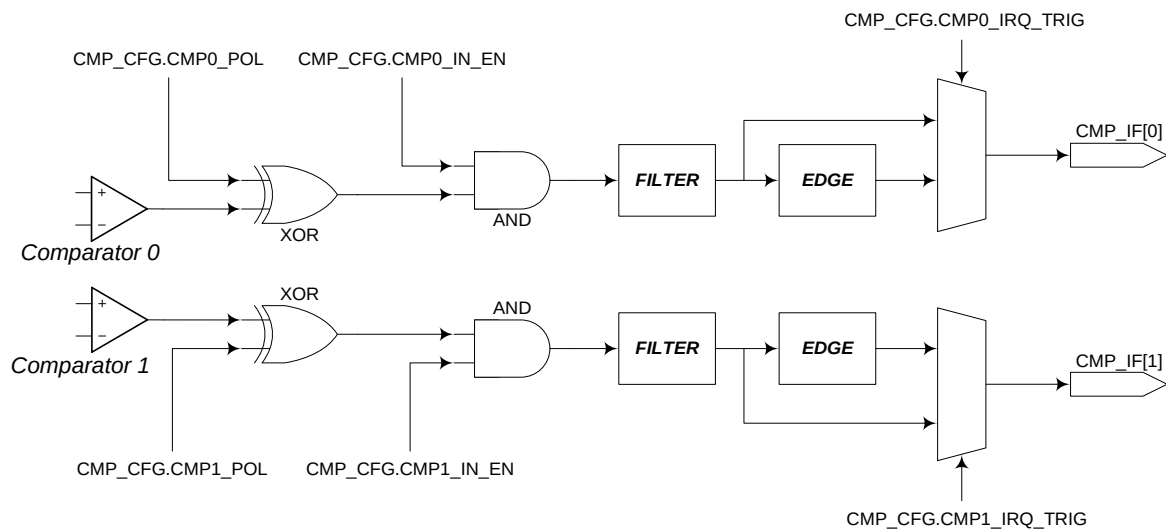
图 17-2 比较器控制及中断产生逻辑
