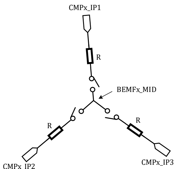
图 4-2 BEMFx_MID 信号
