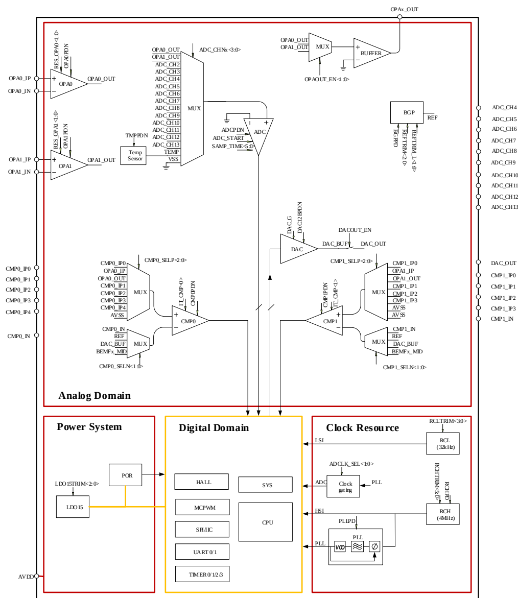
图 4-1 模拟电路功能框图
