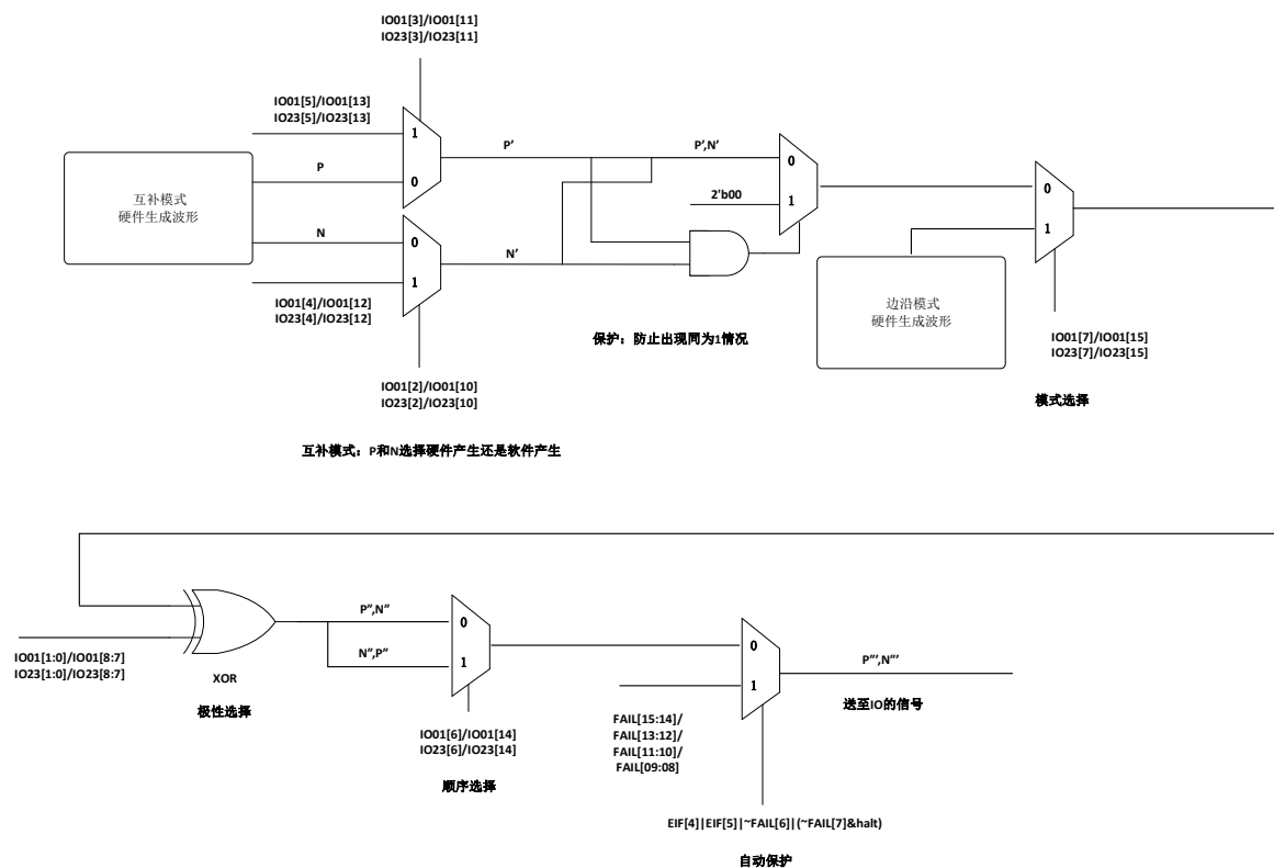
图 12-6 IO Driver 模块数据流程图
