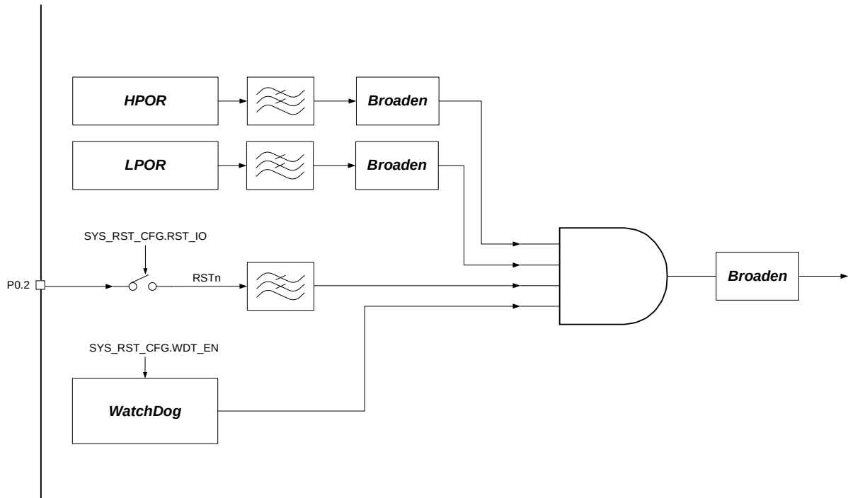
图 5-2 复位架构
