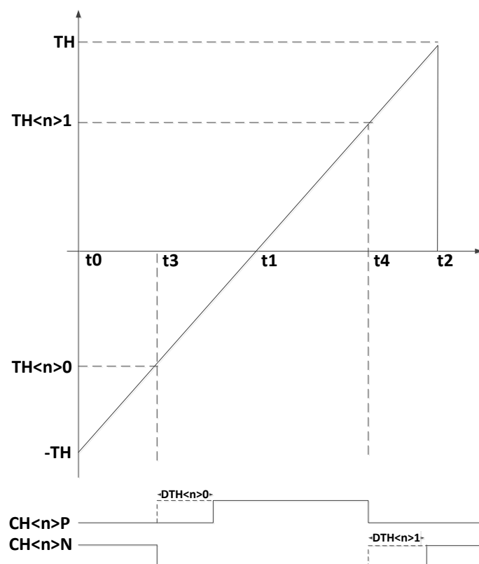
图 12-7 MCPWM 时序 TH&lt;n&gt;0 和 TH&lt;n&gt;1-中心对齐模式
