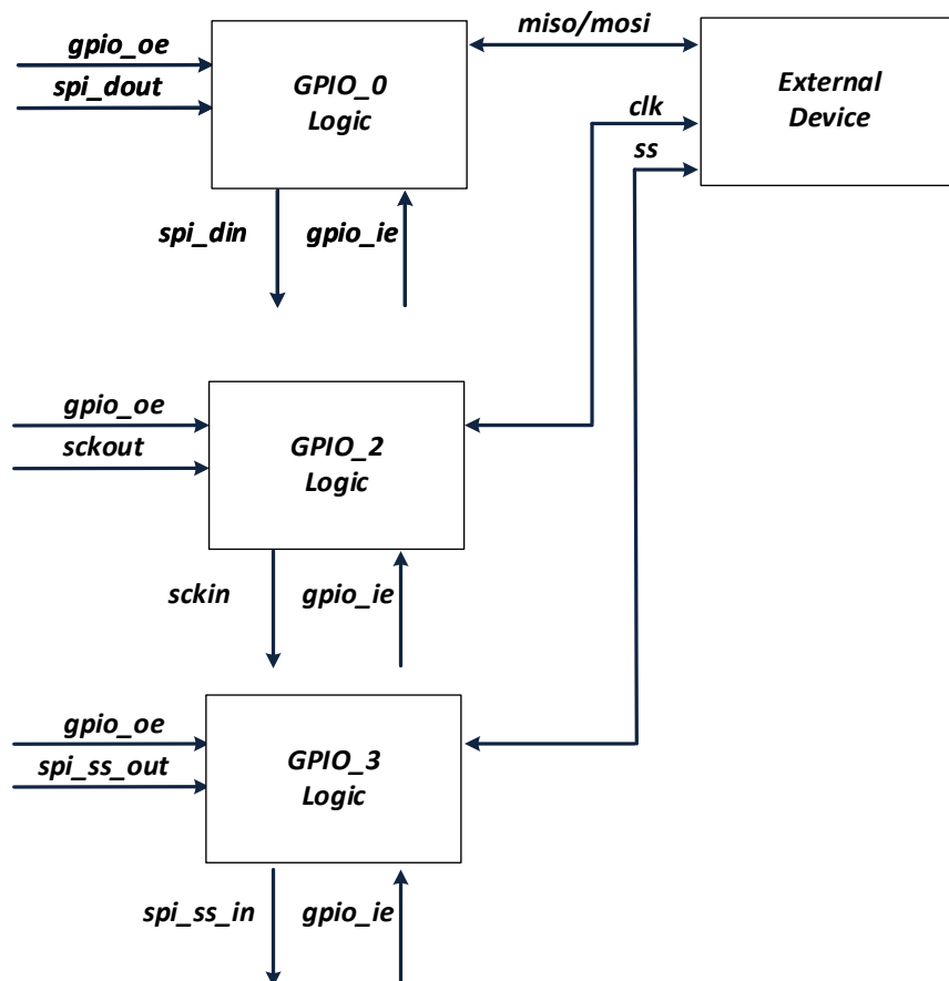
图 16-3 SPI 接口半双工模式互连框图
