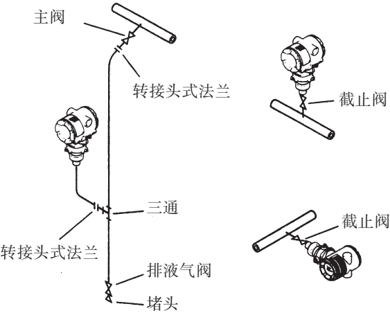
图 5.2 引压管连接示例
