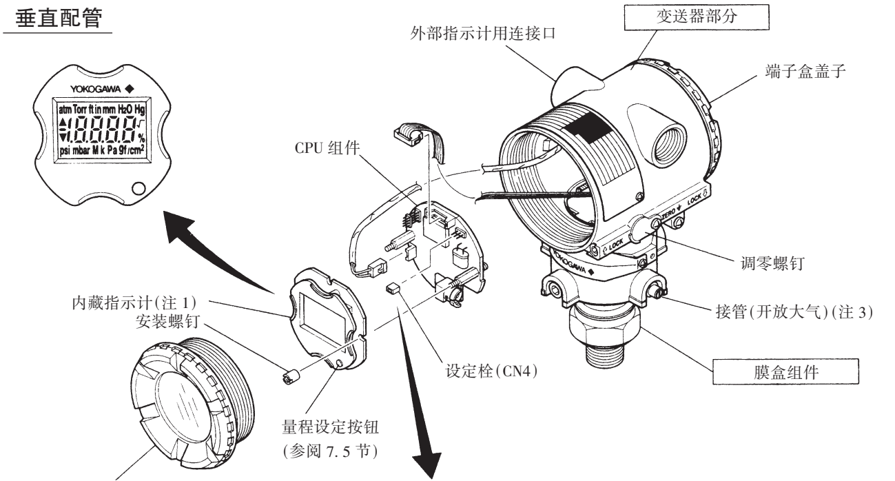
图 3.1 部件名称
