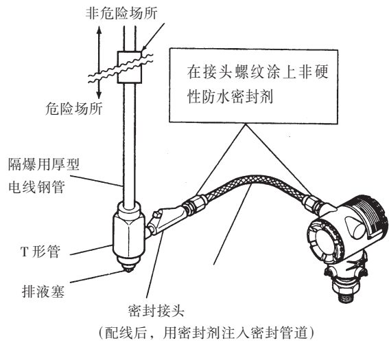
图 6. 4. 2c 用隔爆金属导线管的典型配线
