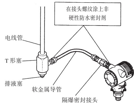
图 6. 4. 2b 用隔爆密封接头的典型配线
