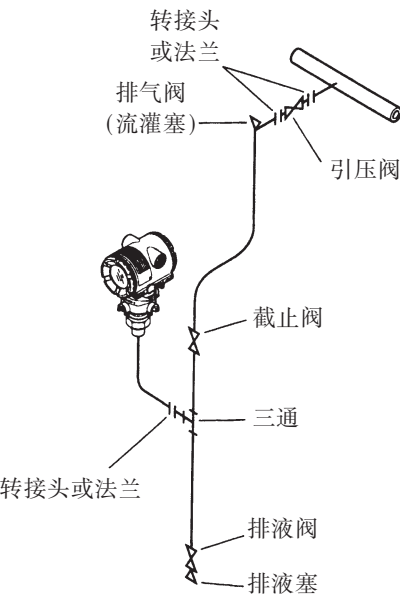
图 7.1 液体流测量(表压变送器)
