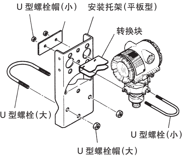
图 2.1.1 变送器安装部件
