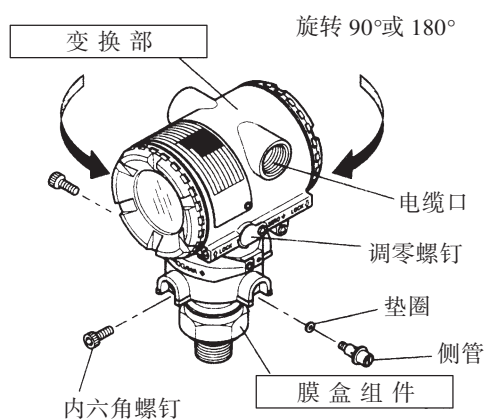
图 4.3 旋转变送部
