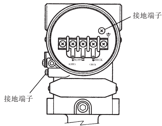
图 6. 5 接地端子
