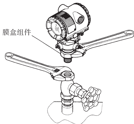
图 4.2.3 膜盒组件
