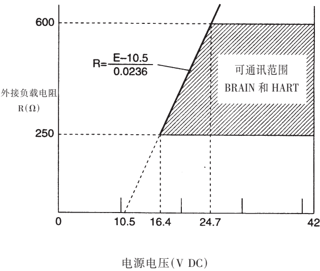
图 6. 6 电源电压与外接负载电阻之间关系
