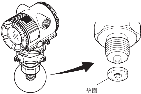
图 4.2.2 垫圈
