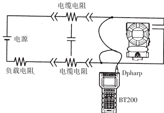
图 8.1.2 回路
