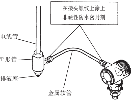
图 6.4.2a 典型金属软管配线
