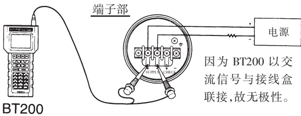
图 6.3.3 BT200 的连接
