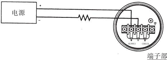
图 6.3.1 电源连接
