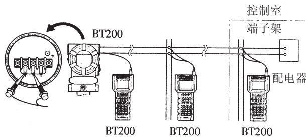
图 8.1.1 BT200 的连接
