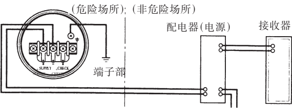
图 6.4.1a 变送器与配电器的连接
