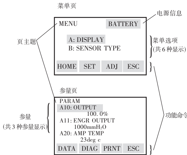
图 8.2.1 BT200 面图
