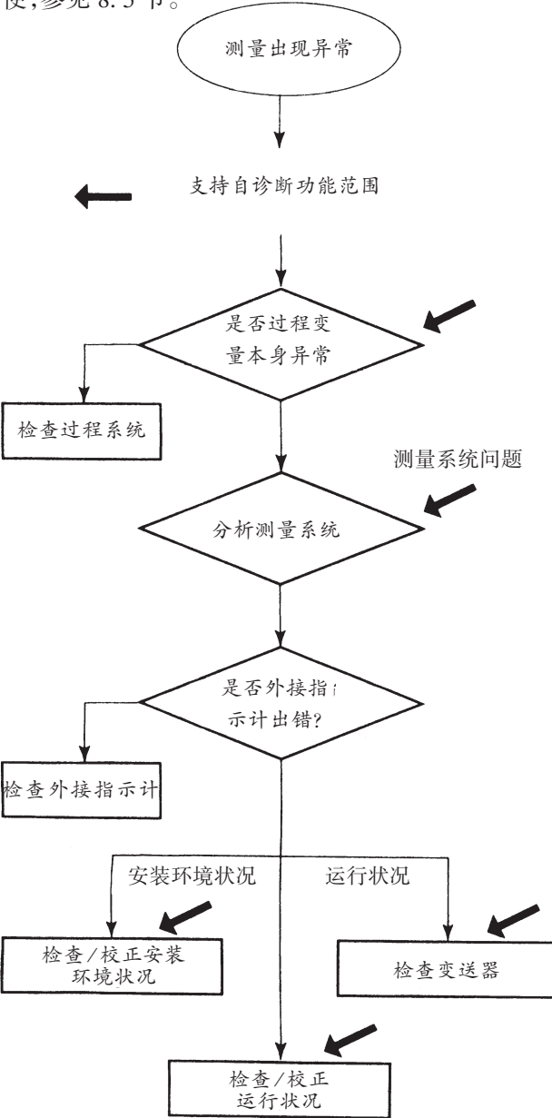
图 9.5.1 基本流程及自诊断
