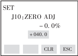
将设定值改为实测值 (40.0%) 按 ENTER 键 两次, 40.0% 对应输出 为 10.4mA DC。
