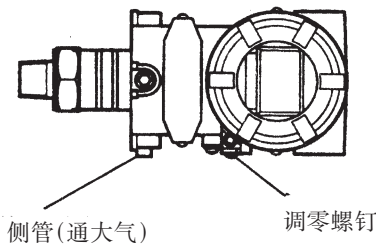
图 5.1.1 水平配管连接
