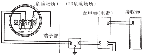
图 6.4.1b 变送器与配电器的连接
