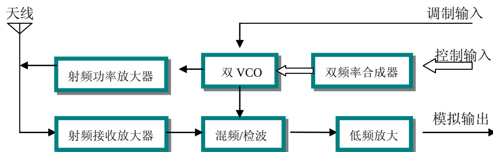
泰达鑫系列无线数传电台方框图（音频传输）
