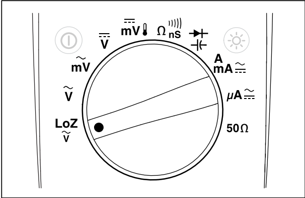
图 3.旋转开关
