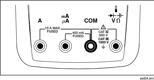
图 4.输入端子
