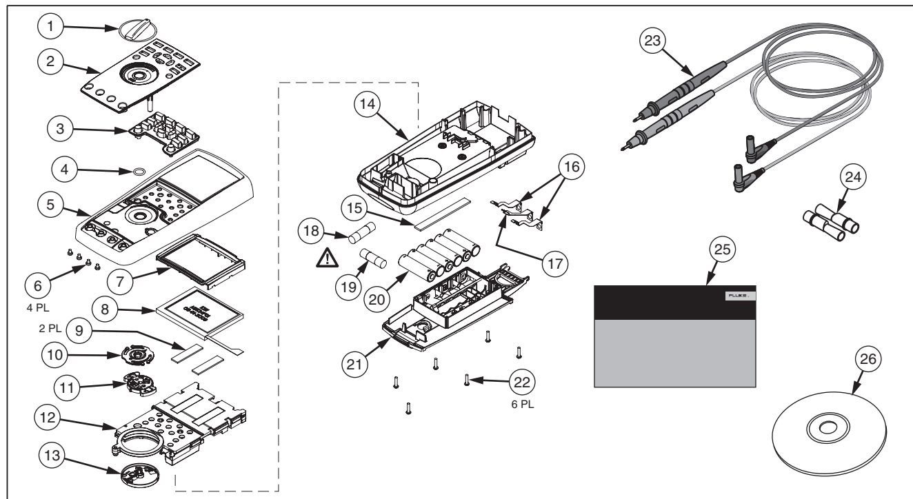
图 31. 可更换零件
