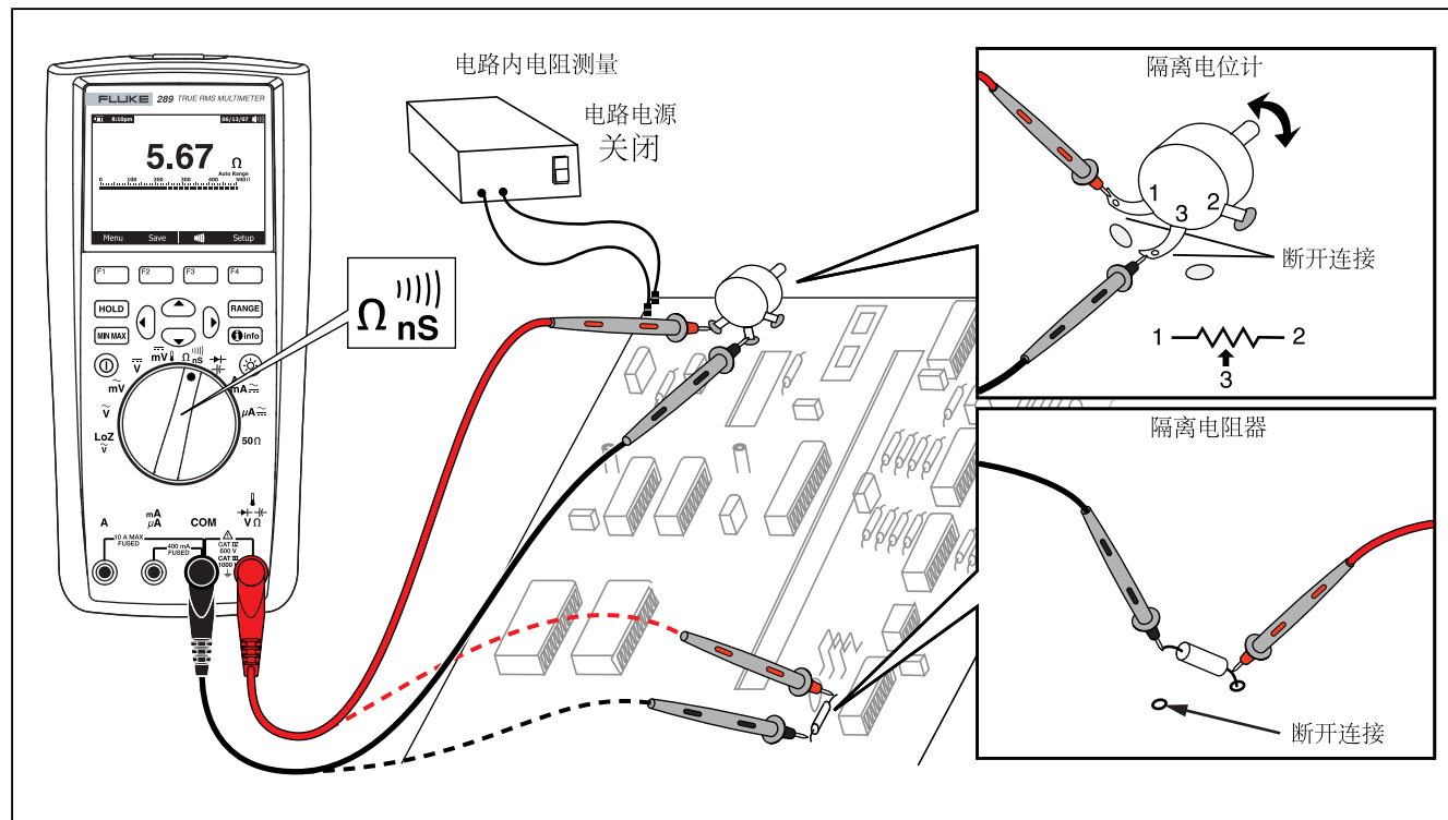
图 15.电阻测量
