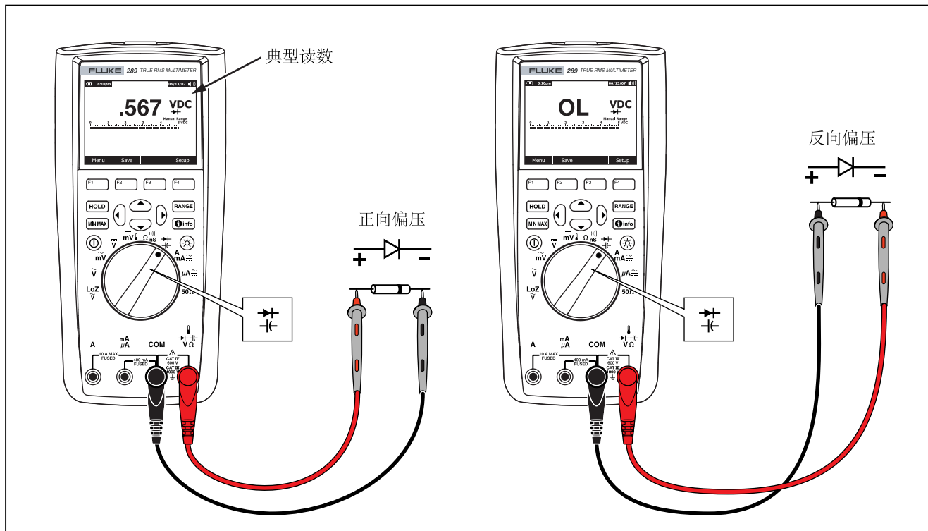
图 20.二极管测试
