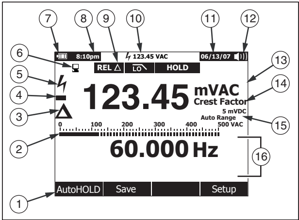
图 2. 显示屏特性
