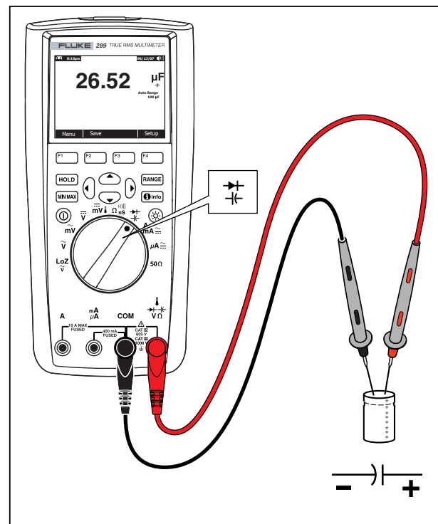
图 19. 电容测量
