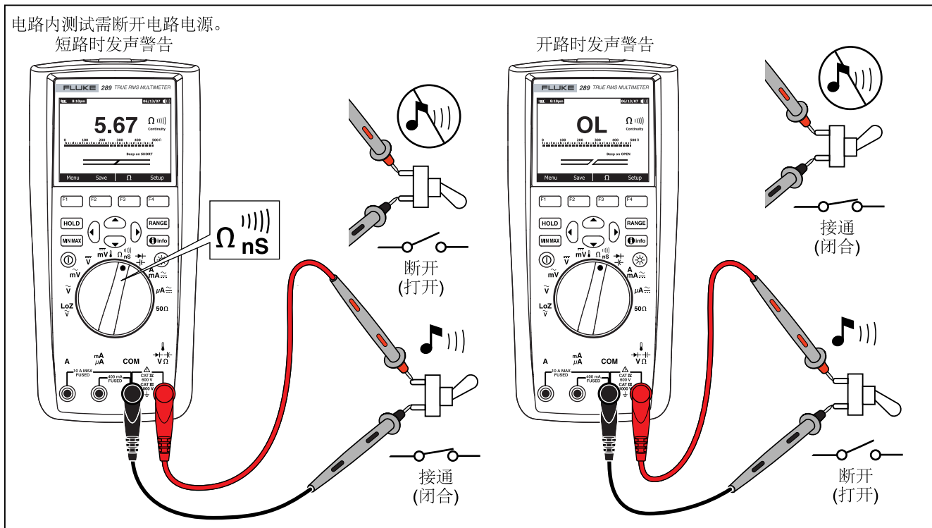
图 17.通断性测试
