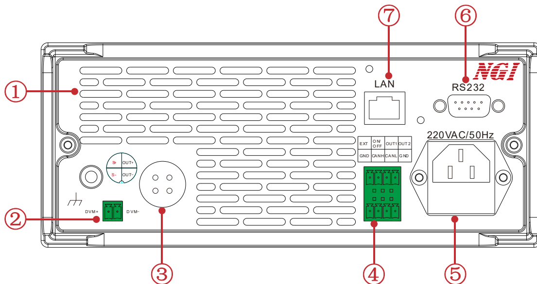
图 3-8 后面板
