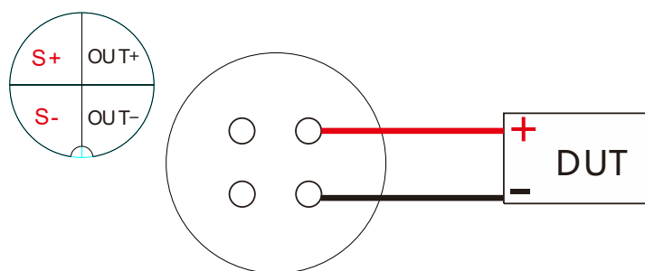
图 3-14 后面板两线本地测量
