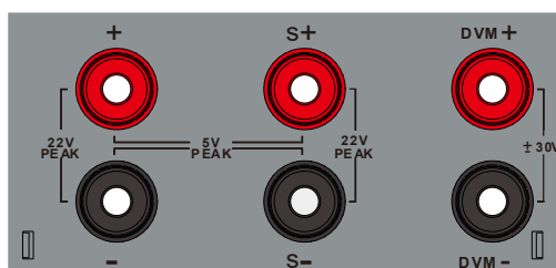
图 3-7 前面板通道端子
