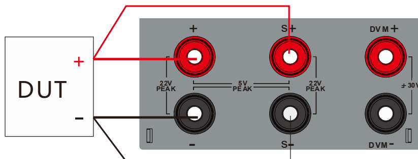
图 3-15 前面板四线远端测量
