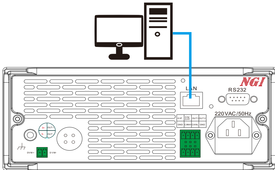
图 3-12 接线图
