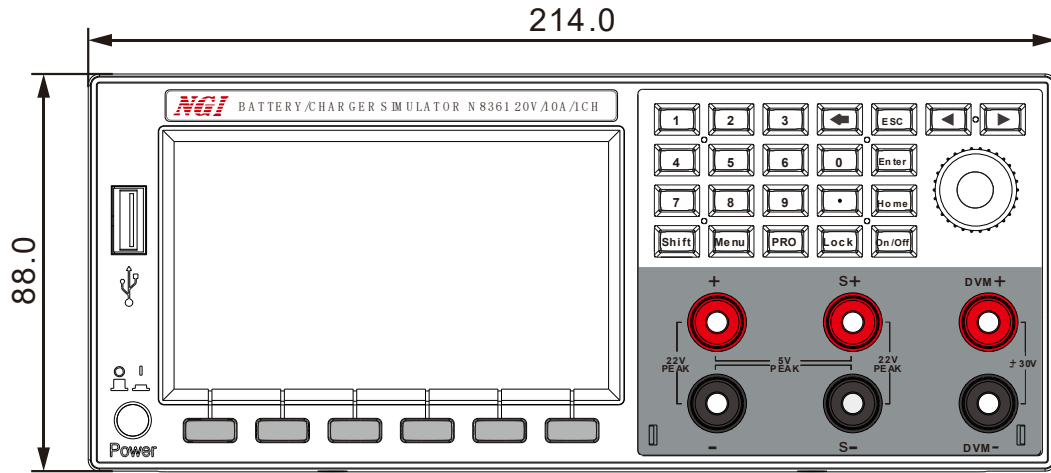
图 3-1 前面板尺寸
