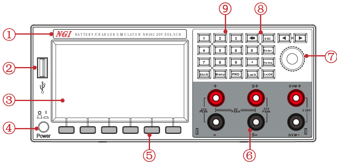
图 3-4 前面板
