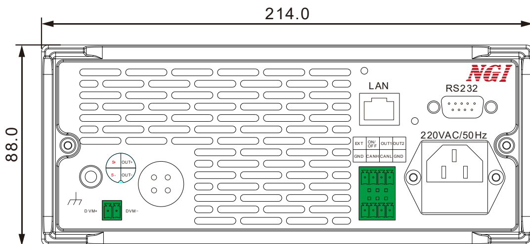
图 3-3 后面板尺寸
