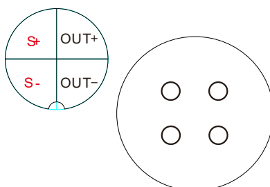
图 3-9 通道端口
