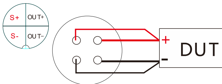
图 3-16 后面板四线远端测量
