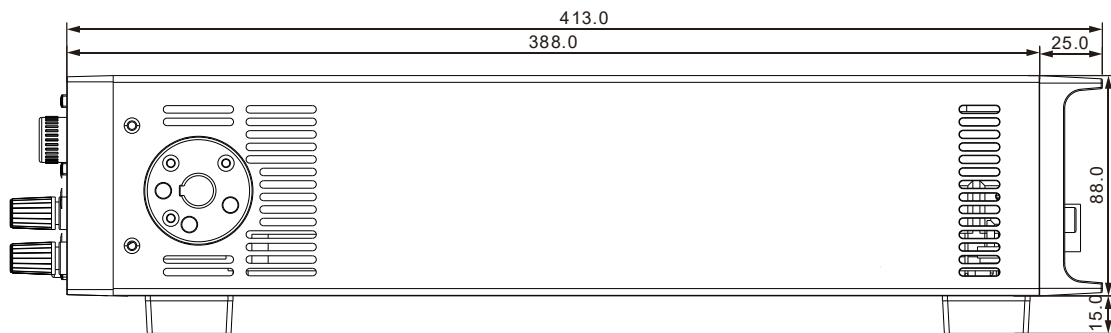
图 3-2 机箱侧视尺寸
