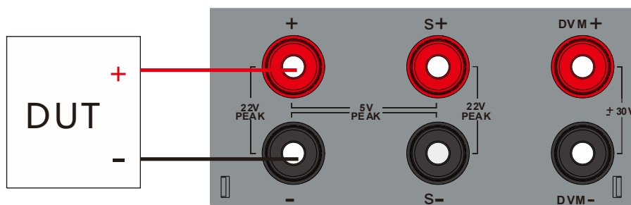
图 3-13 前面板两线本地测量
