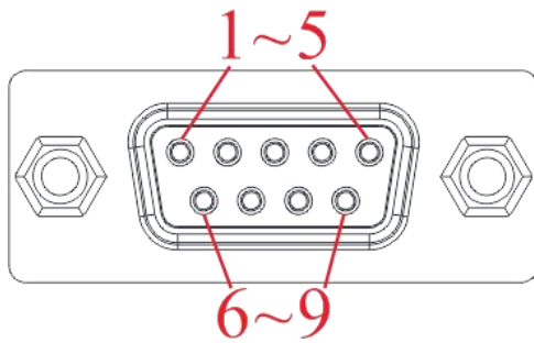
图 3-11 RS232 引脚标识
