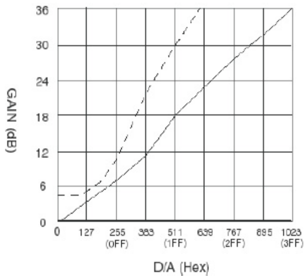
图 4 MVC610DAC-GE110 增益控制曲线
