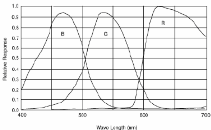
图 1 MVC610DAC-GE110 的光谱曲线
