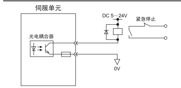
继电器回路示例
