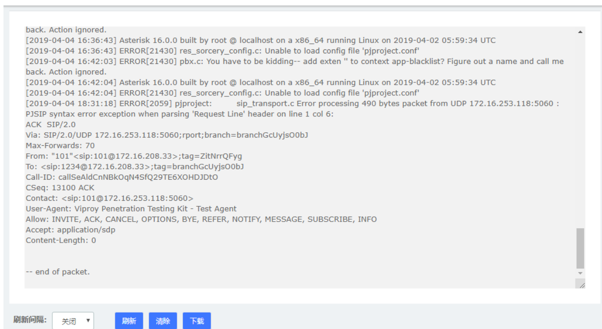
图 7-3 Asterisk 日志
