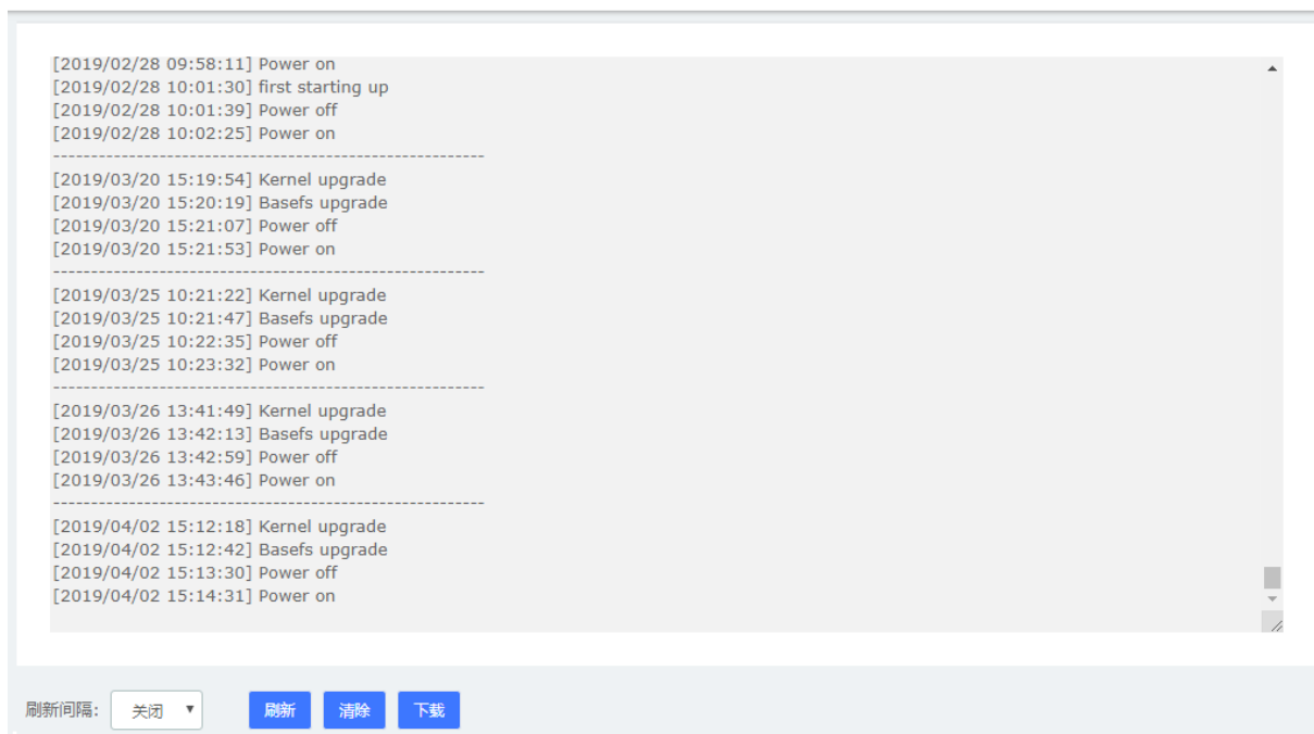
图 7-2 系统日志
