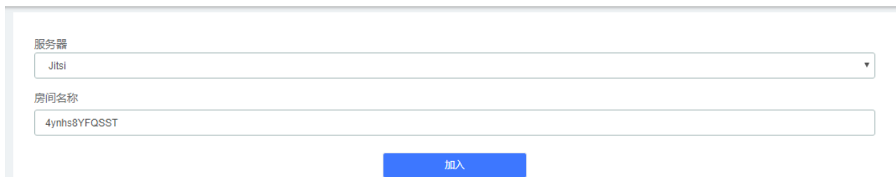
图 6-2 视频会议
