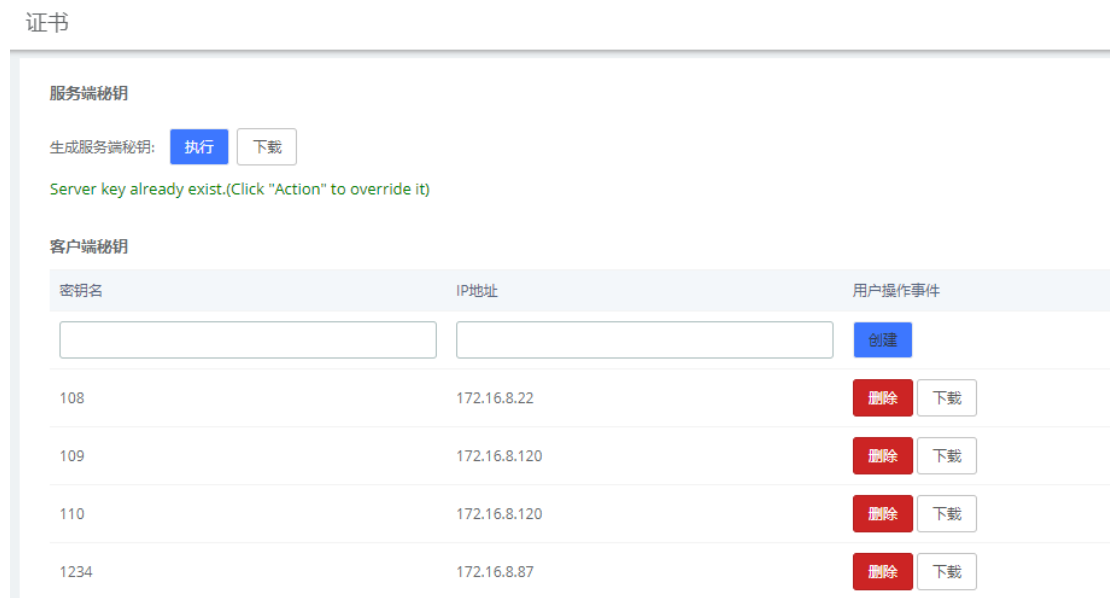
图 2-19 证书设置
