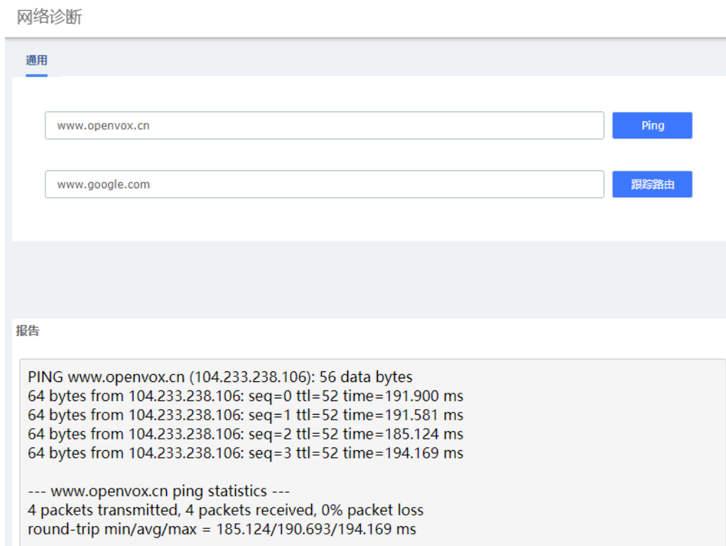
图 2-48 网络诊断
