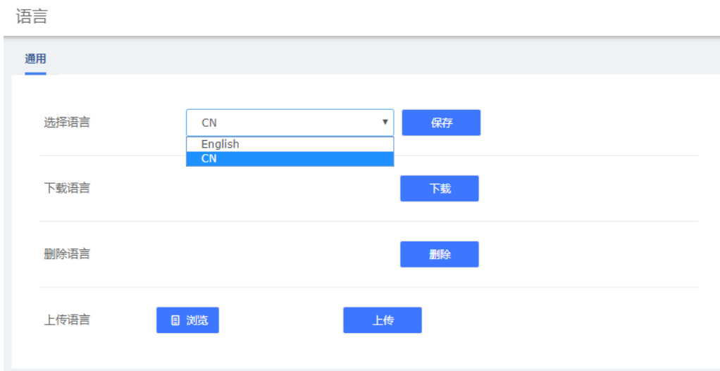
图 2-49 语言
