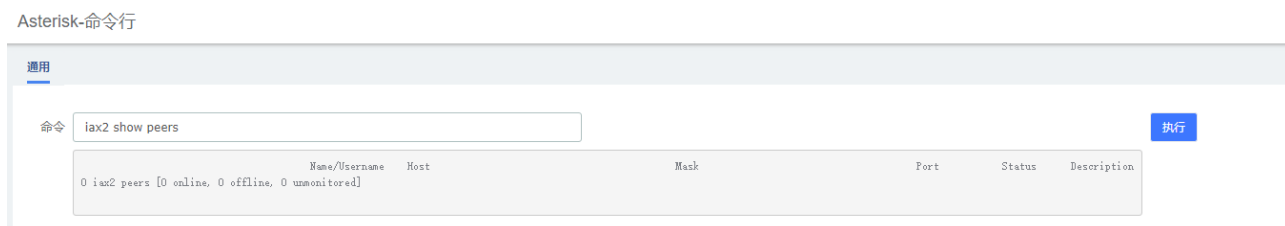
图 3-108 Asterisk-命令行
