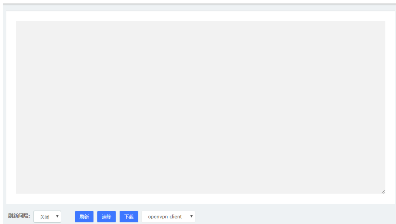
图 7-6 VPN 日志
