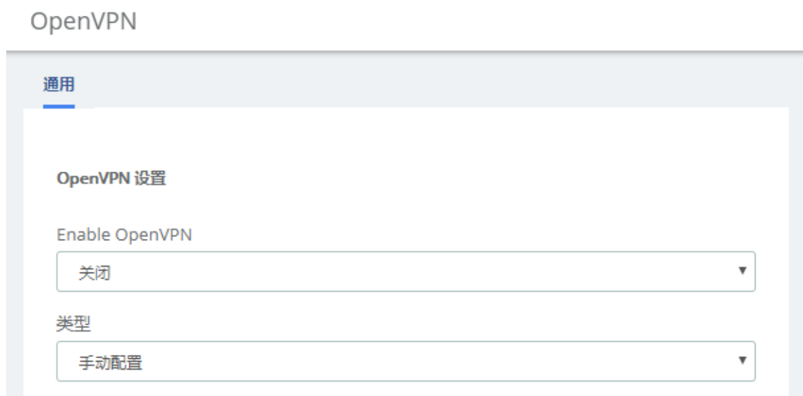
图 2-7 OpenVPN
