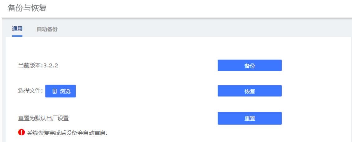
图 2-37 备份与恢复
