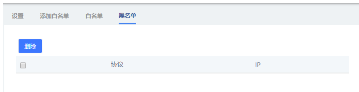
图 2-25 Fail2Ban 黑名单
