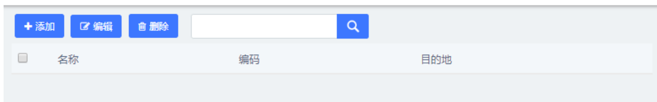
图 3-69 语言
