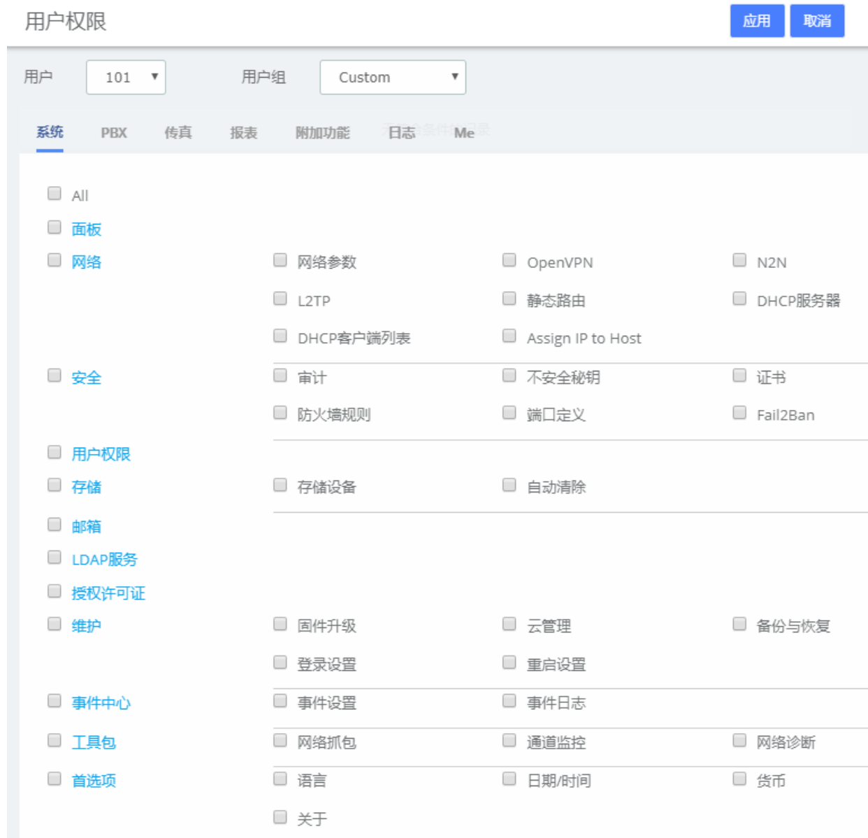
图 2-27 新建用户
