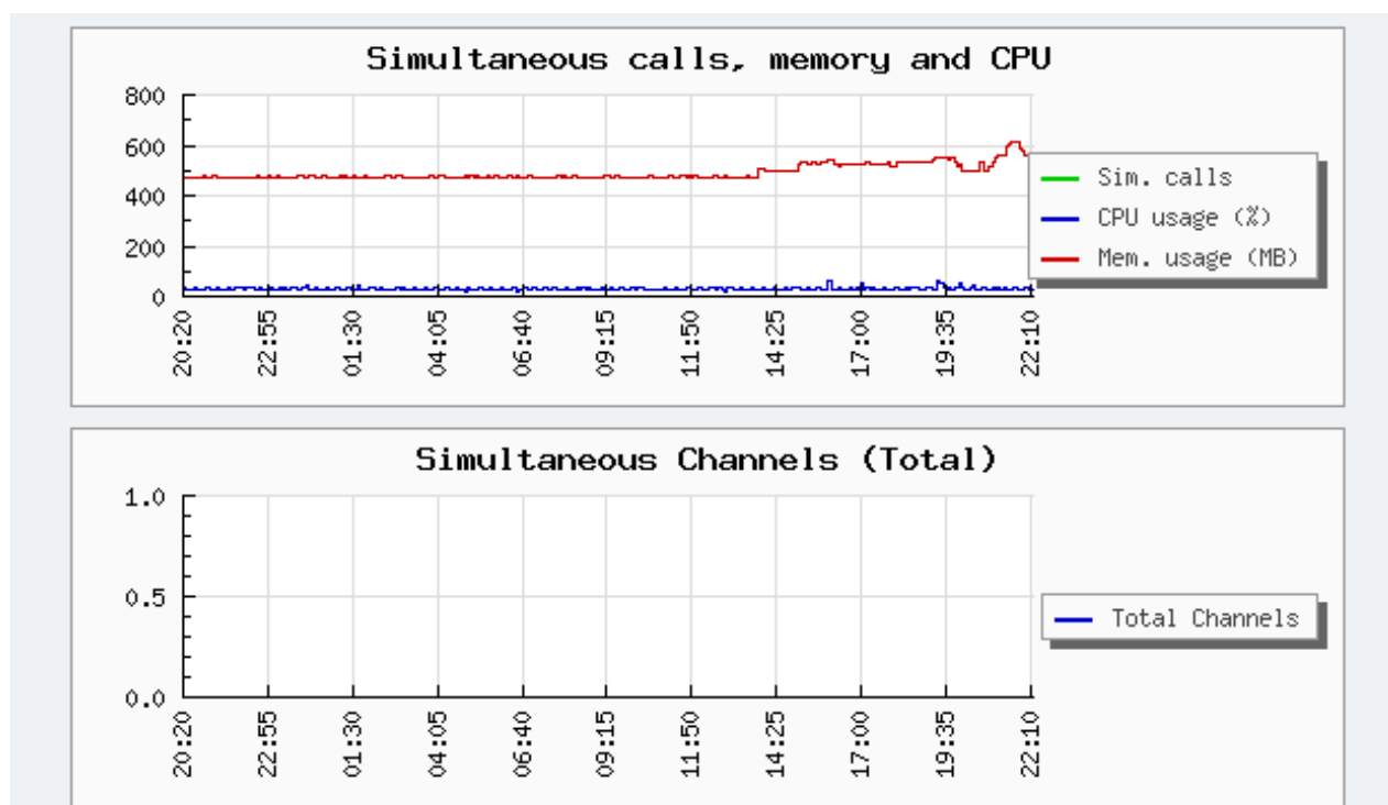
图 5-2 通道使用量
