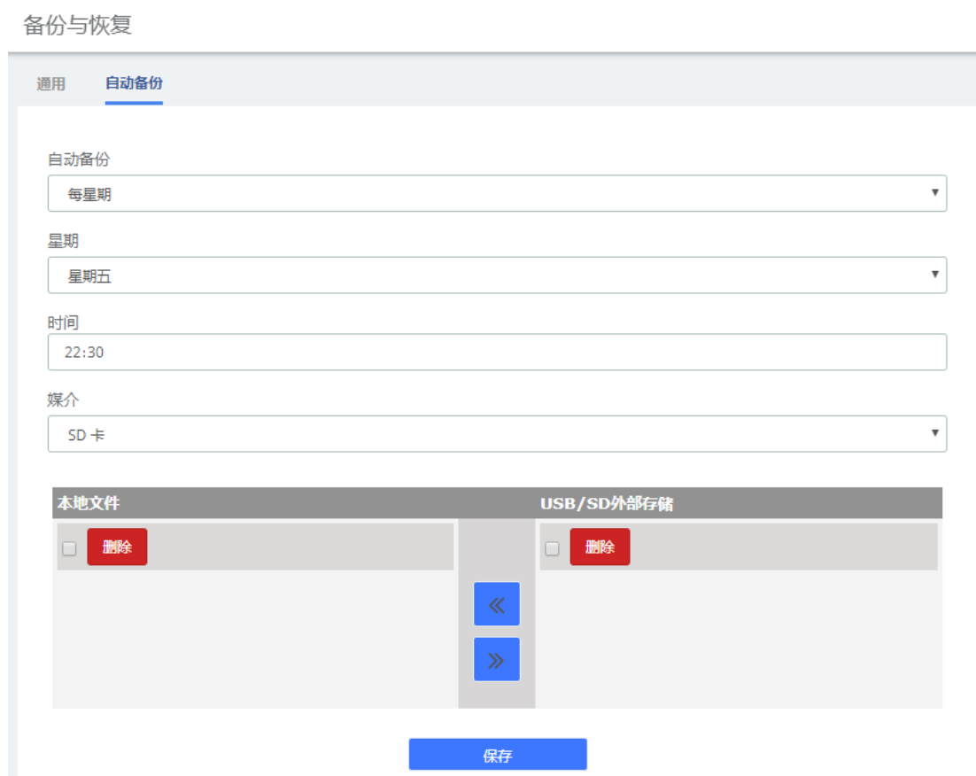
图 2-38 自动备份
