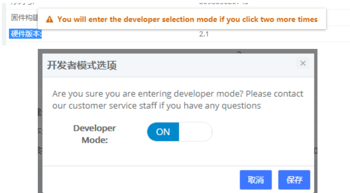
图 2-53 开发者模式
