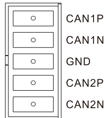
图 3-13 CAN 引脚标识
