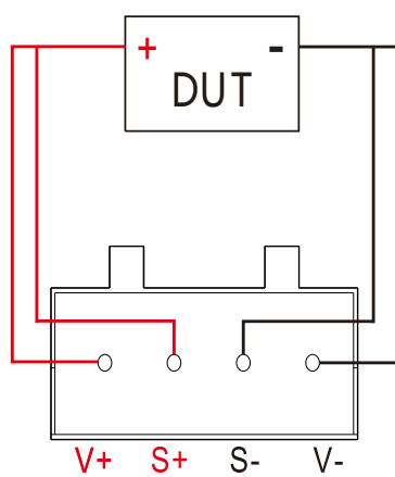
图 3-16 接线图
