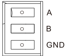
图 3-11 RS485 引脚标识
