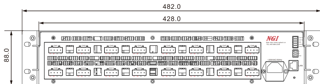
图 3-3 后面板尺寸
