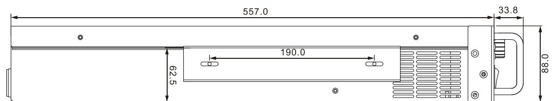
图 3-2 机箱侧视尺寸
