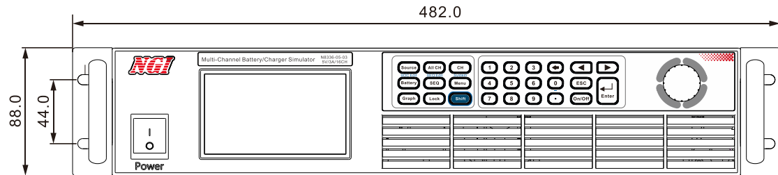
图 3-1 前面板尺寸
