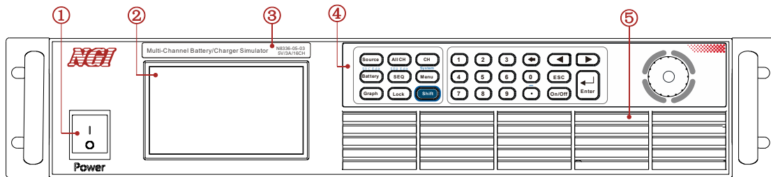
图 3-4 前面板
