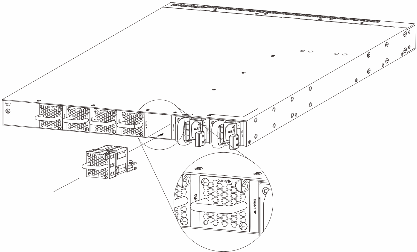
Figure 3-13 Installing a Fan Module
