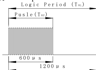
图 4 低电平脉宽、逻辑周期宽度
