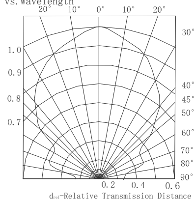
f) Directivity
