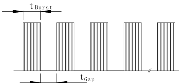
图 2 脉冲宽度和间隔时间 Figure 2 Burst Length and Gap Time
