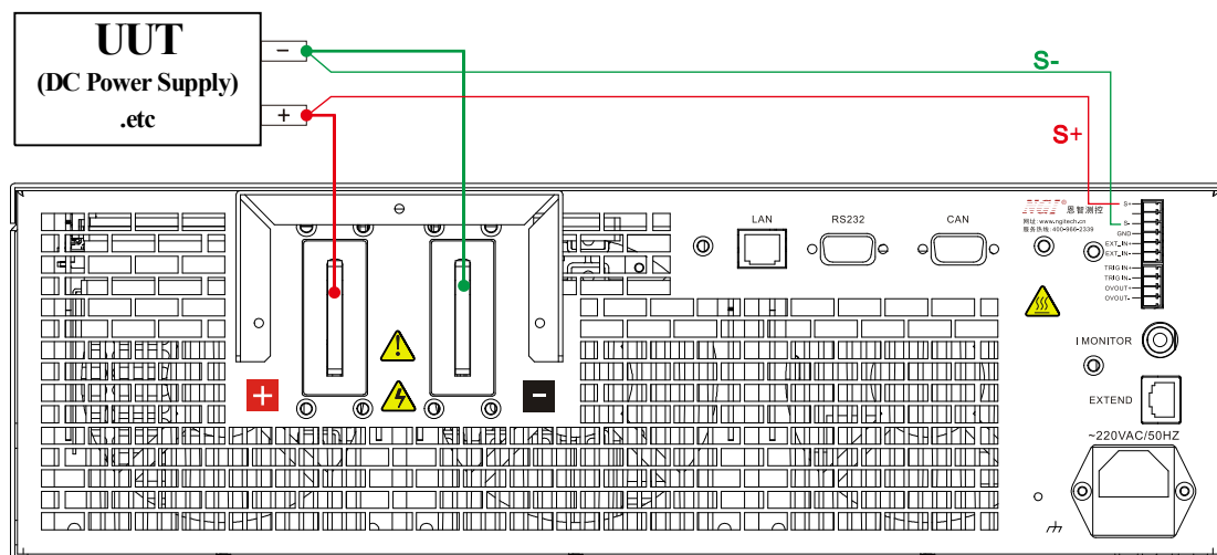
图 3-7 远端采样连接
