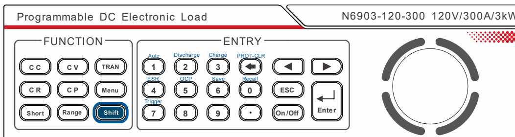
图 5-1 电子负载键盘
