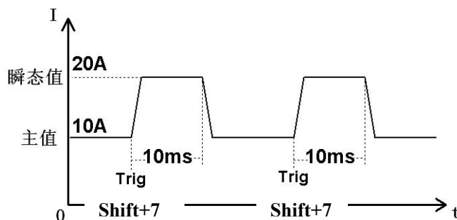
图 4-6 脉冲方式
