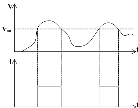
图 4-12 非锁定 V_{on} 带载
