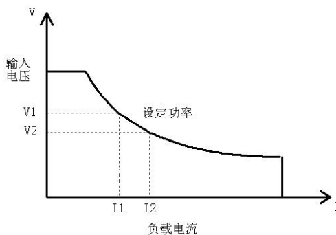
图 4-4 恒功率模式
