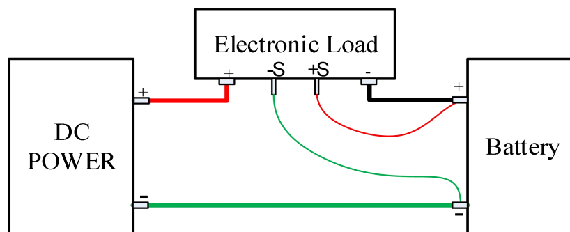
图 4-10 充电测试接线示意图
