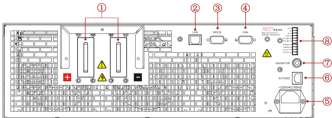
图 3-5 主机后面板
