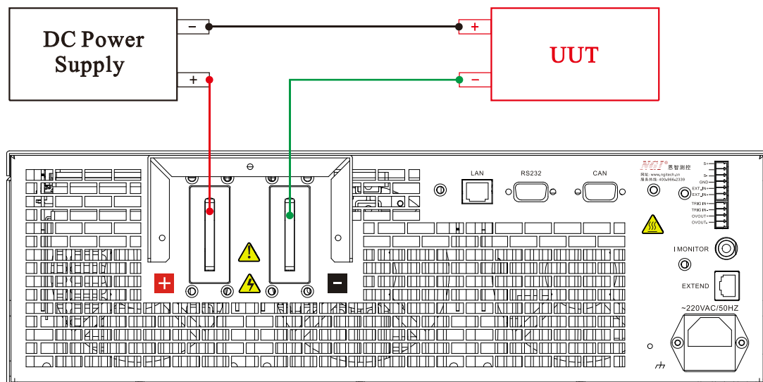
图 3-9 低电压操作
