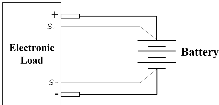
图 6-16 电池内阻测试连线图
