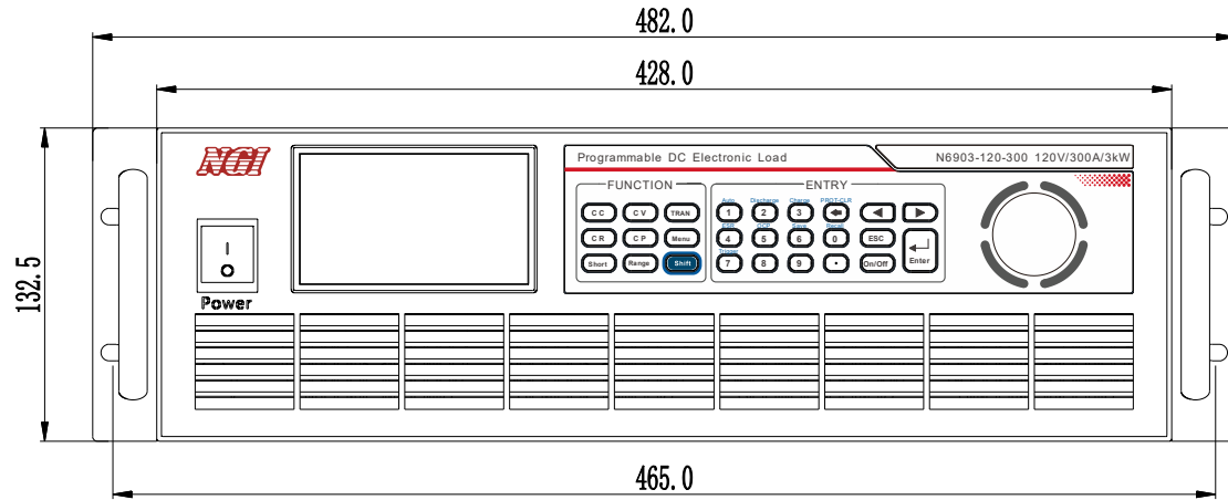
图 3-1 主机正面尺寸图 (mm)
