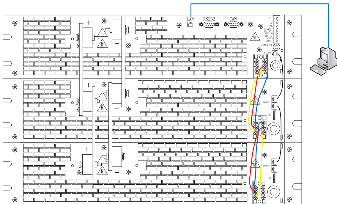
图 3-10 多机并联图
