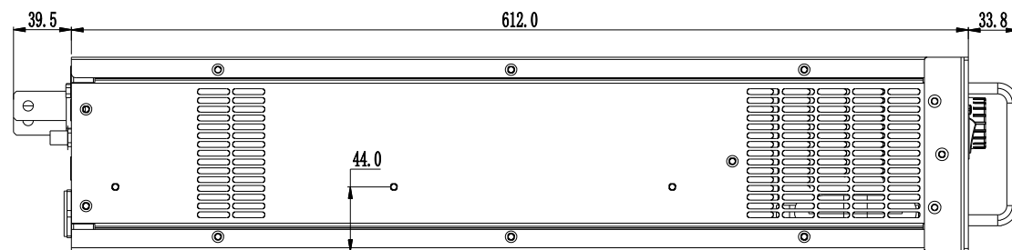
图 3-2 主机侧面尺寸图 (mm)
