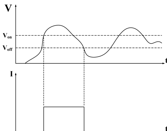
图 4-13 锁定 V_{on} 带载和 V_{off} 卸载
