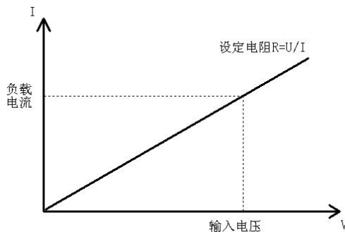
图 4-3 恒电阻模式
