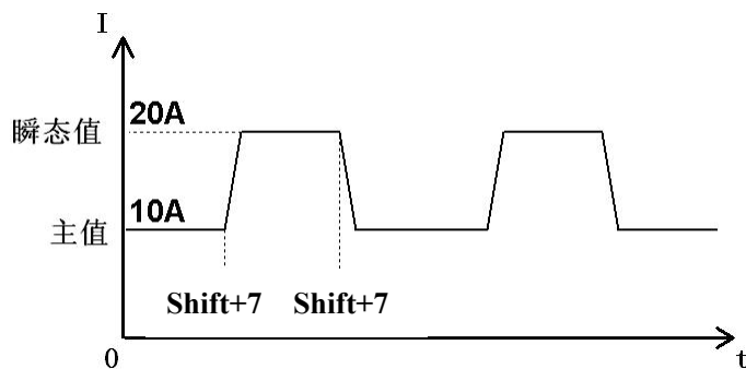
图 4-7 翻转方式
