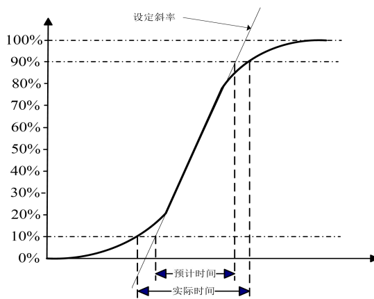
图 4-14 斜率与实际转换时间的关系
