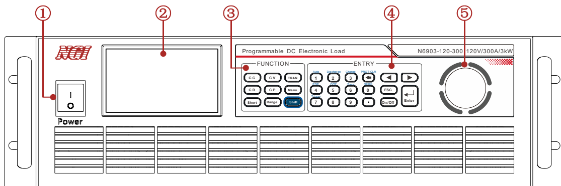
图 3-4 主机前面板
