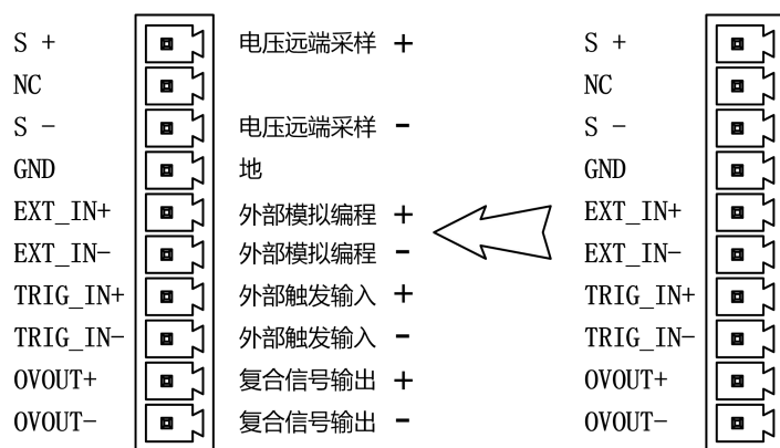
图 3-6 负载控制连接端子
