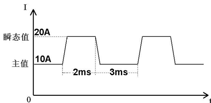
图 4-5 连续方式
