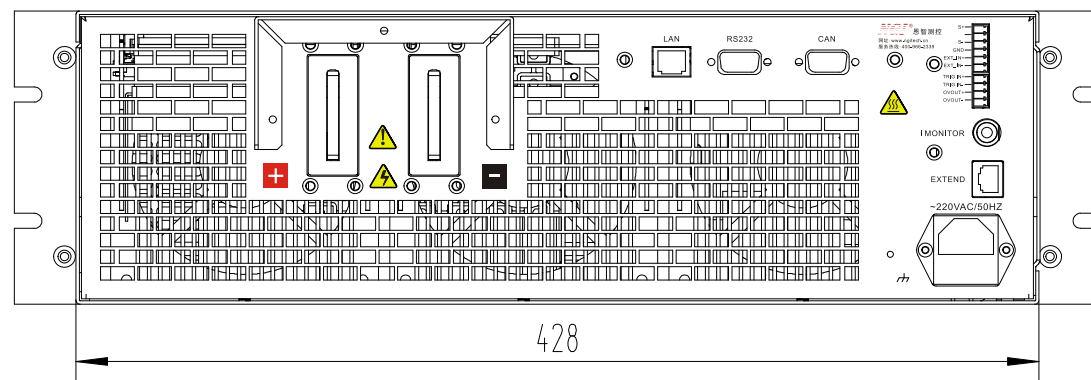
图 3-3 主机后面板尺寸图 (mm)
