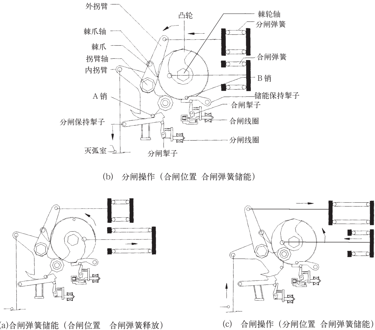
图9 弹簧操作机构的结构及工作原理图
