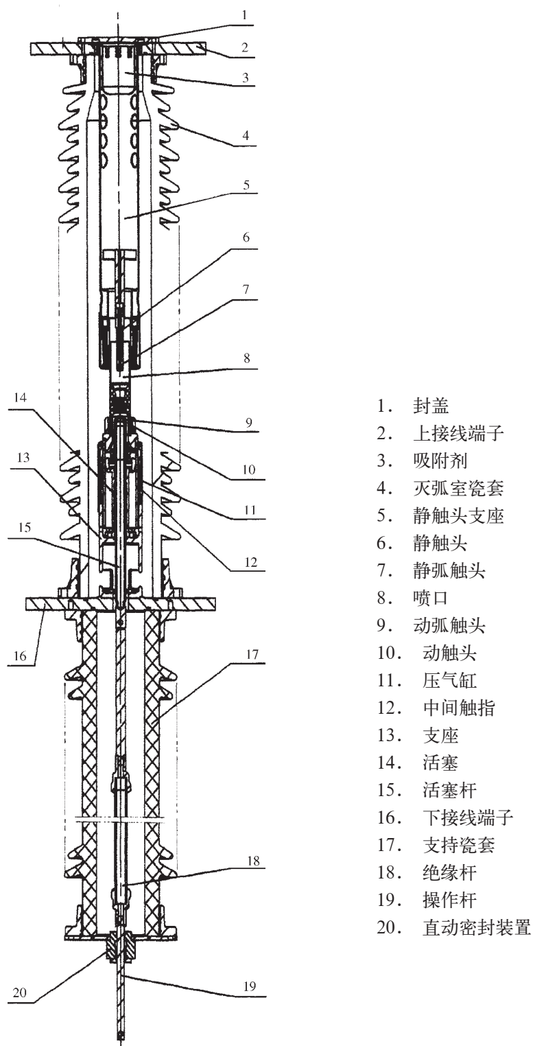
图 6 单极断路器结构图
