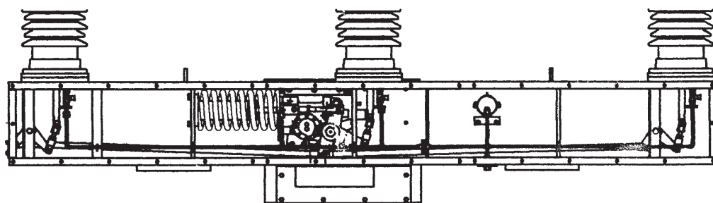
图 8 传动系统结构图
