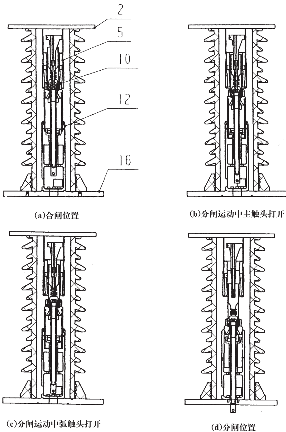
图7 自能灭弧室的开断过程
