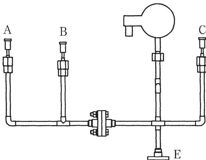
图 10 SF6 气体系统图
