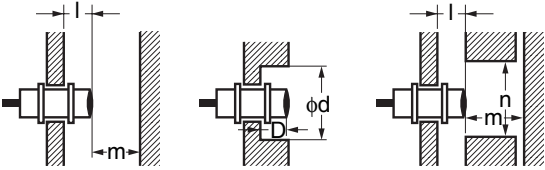
周围金属的影响 数值表示使用附件螺母时／不使用附件螺母时。(单位：mm)
