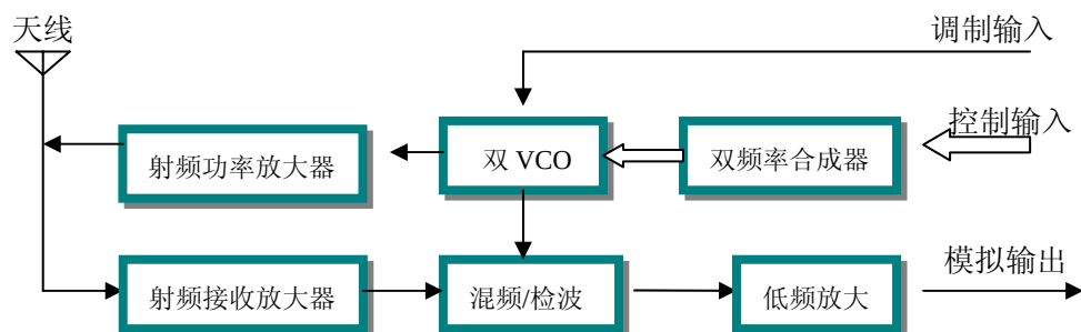
泰达鑫系列无线数传电台方框图（音频传输）
