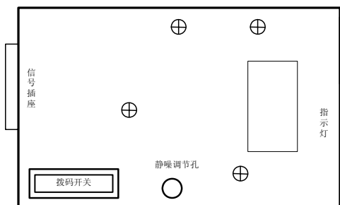
底壳安装孔位图 (可依此位置配散热片) 单位: mm
