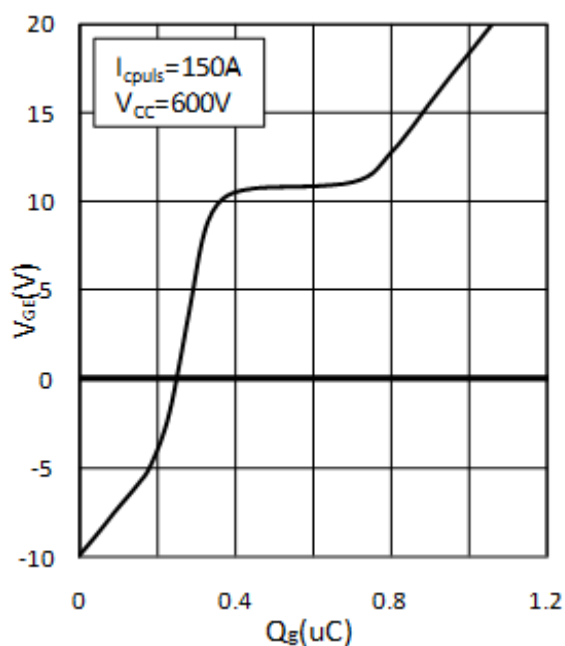
图 13 门极电荷特性
