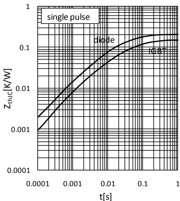
图 15 瞬态热阻
