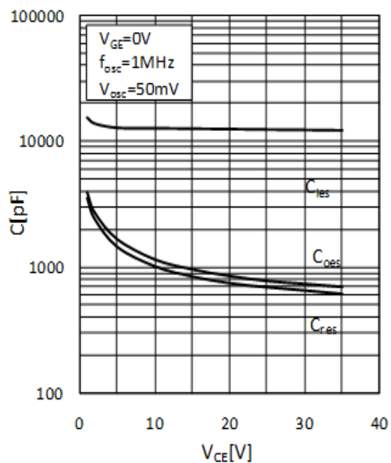
图 14 电容和集-射极电压
