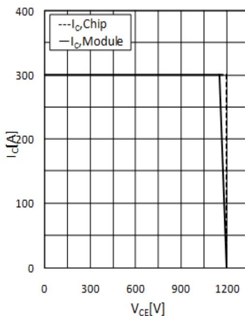
图 16 反偏安全工作区
