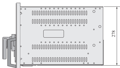
【抽屉式软起动器侧视图】
