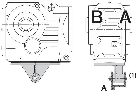
图 9: 斜齿轮 - 伞齿轮减速器的扭矩臂
