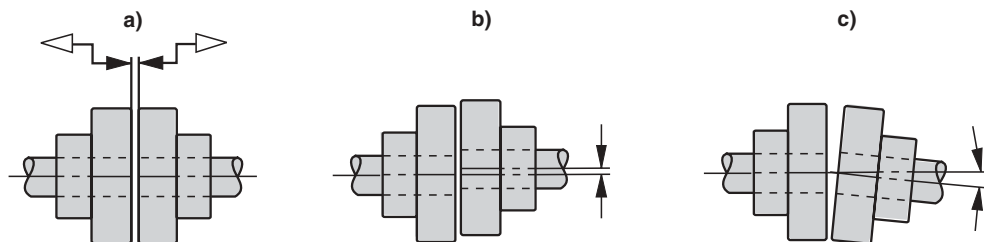
图 7：联轴器装配间距和偏差
