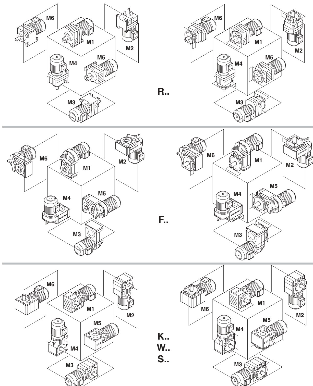
图 14: 图示安装方式 M1 ~ M6
