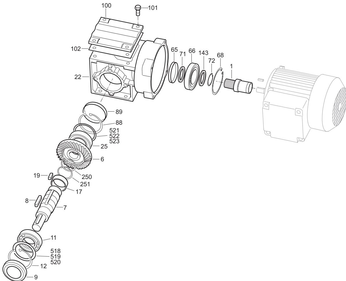
图 5: SPIROPLAN® 减速器的构造原理
