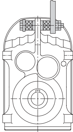
图 8: 平行轴 - 斜齿轮减速器的扭矩臂
