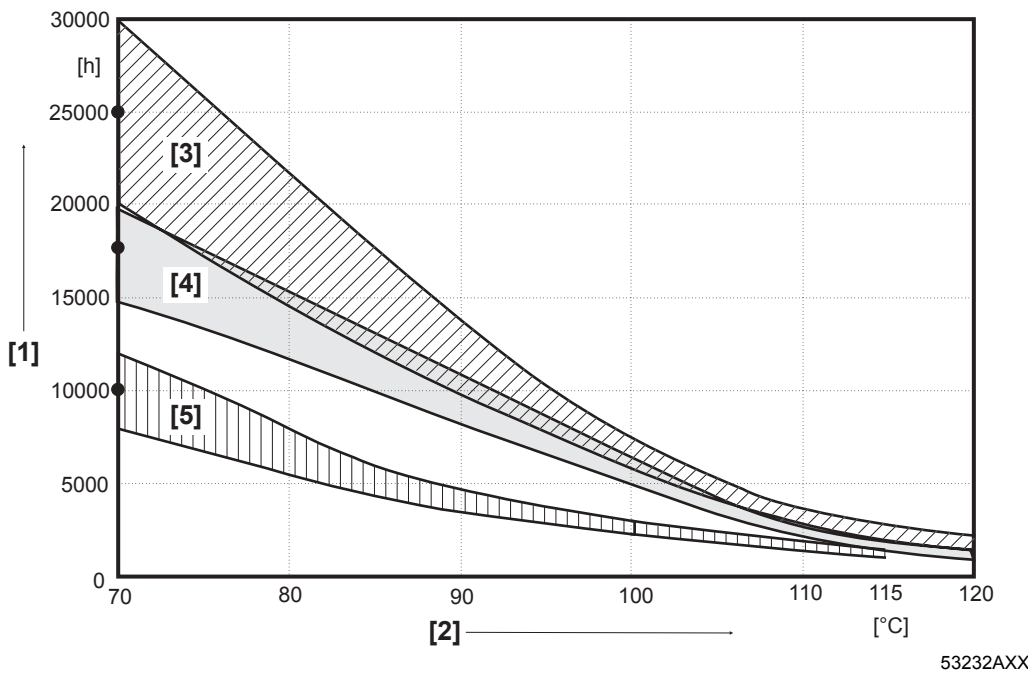
图 13: 适用于正常环境条件下标准减速器的更换时间间隔
