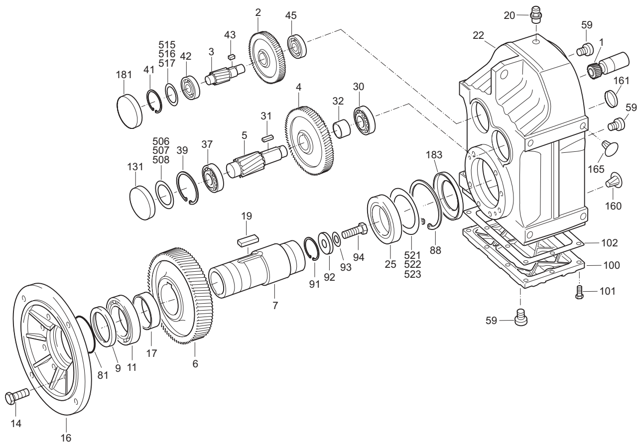
图 2: 平行轴 - 斜齿轮减速器的构造原理
