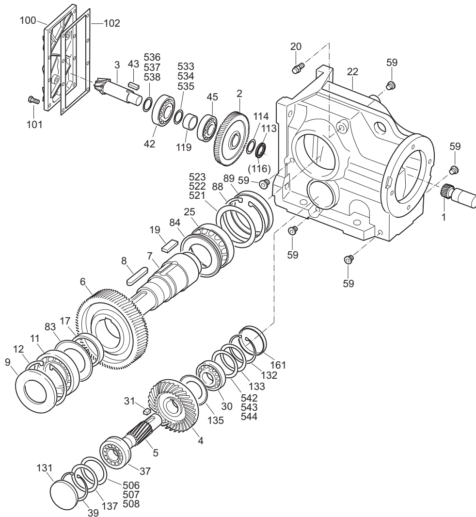
图 3: 斜齿轮 - 伞齿轮减速器的构造原理
