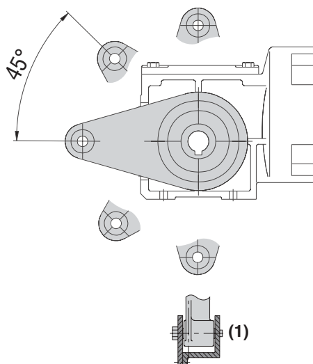
图 11: SPIROPLAN® W 减速器的扭矩臂
