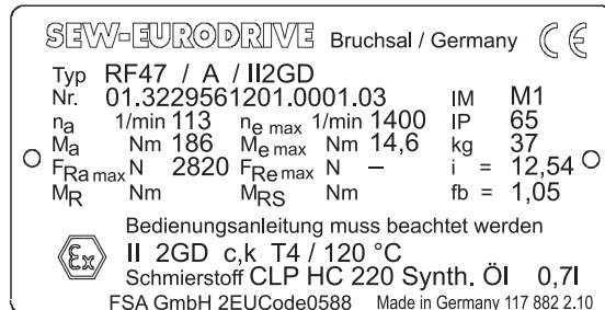
图 6: 铭牌举例
