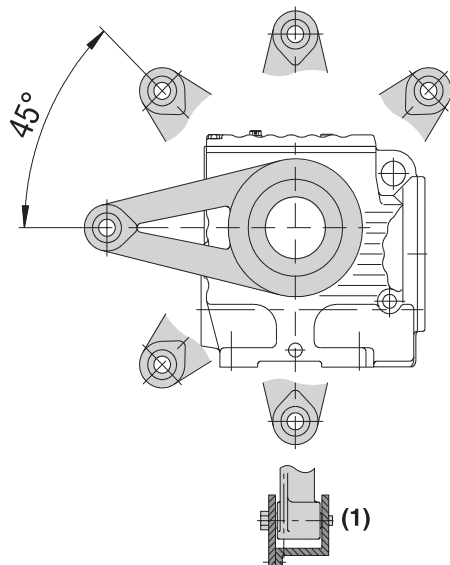
图 10: 斜齿轮 - 蜗轮蜗杆减速器的扭矩臂
