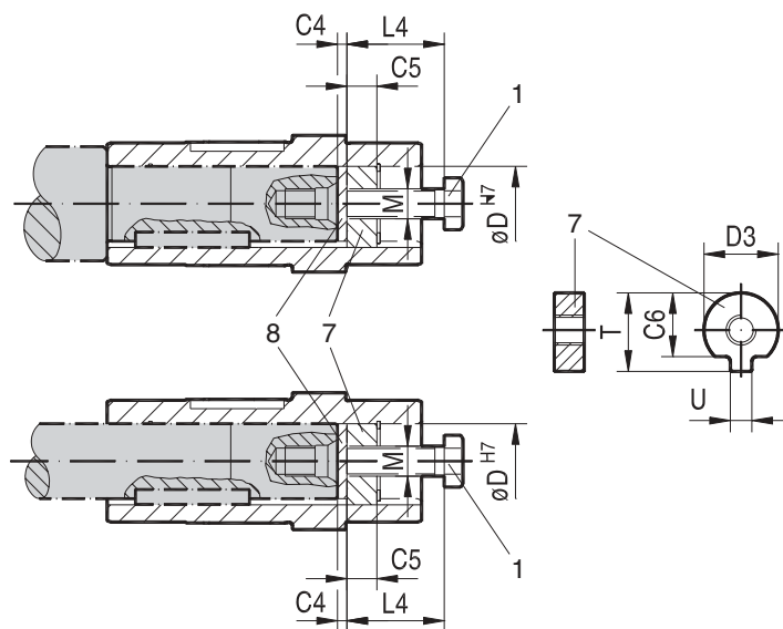
图 12: SEW-EURODRIVE 安装 / 拆卸工具组件
