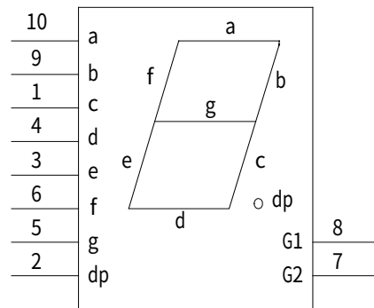
图 5 LG5621AH 元件图
