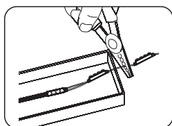
04 剪切模组到所需的数量，并把剪断后的线头做好防水和绝缘处理。
