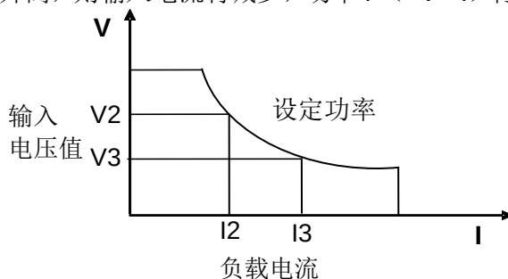
定功率模式 图 3-4 CW 模式电压电流图
