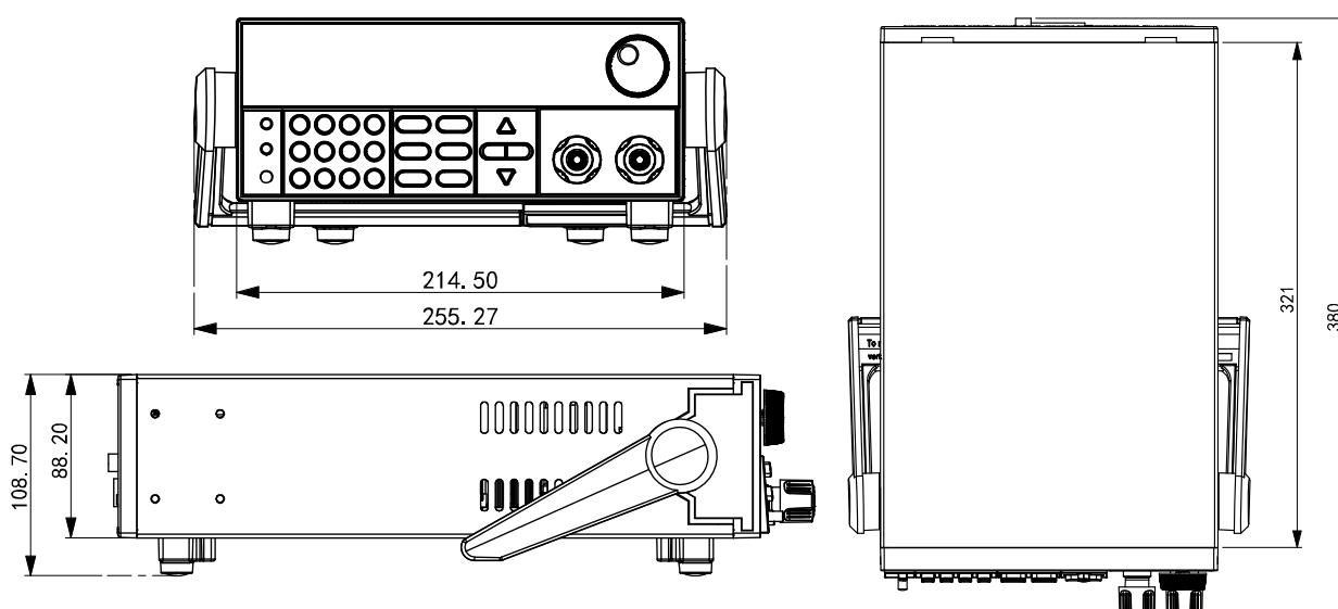
详细尺寸图
