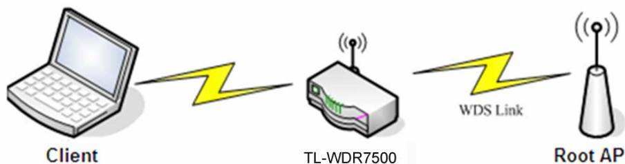
图 5-15 WDS 连接拓扑图
