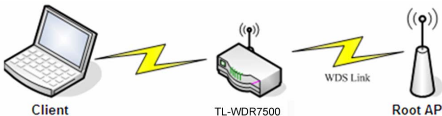
图 5-29 WDS 连接拓扑图
