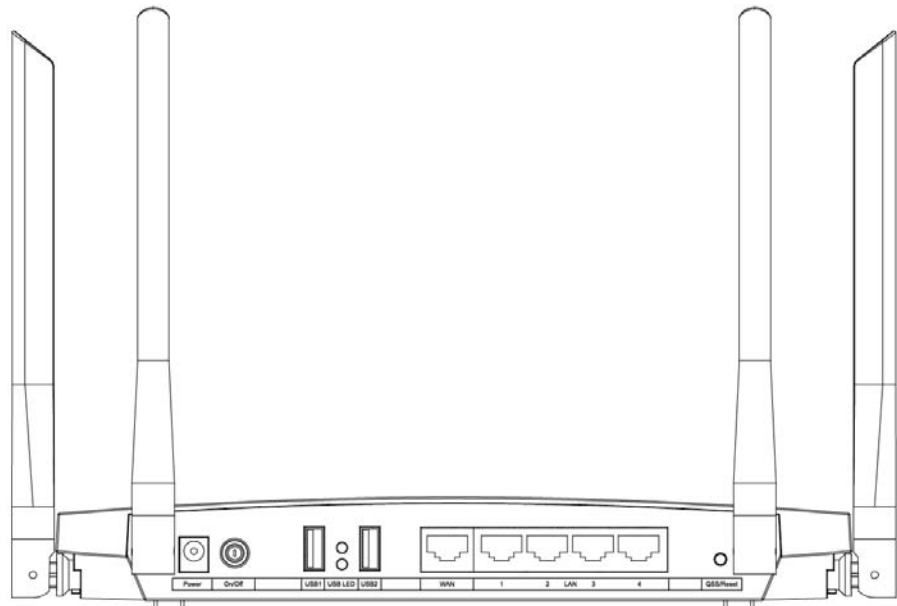
图 3-2 TL-WDR7500 后面板示意图
