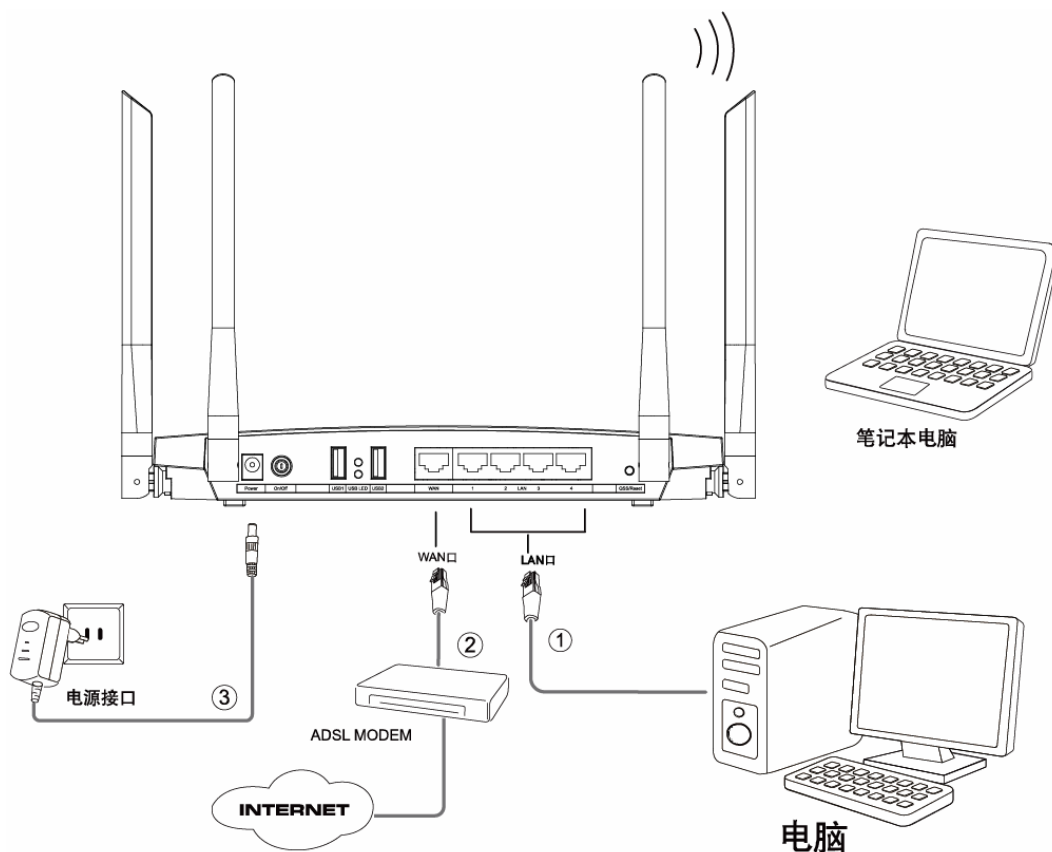
图 4-1 TL-WDR7500 硬件安装示意图
