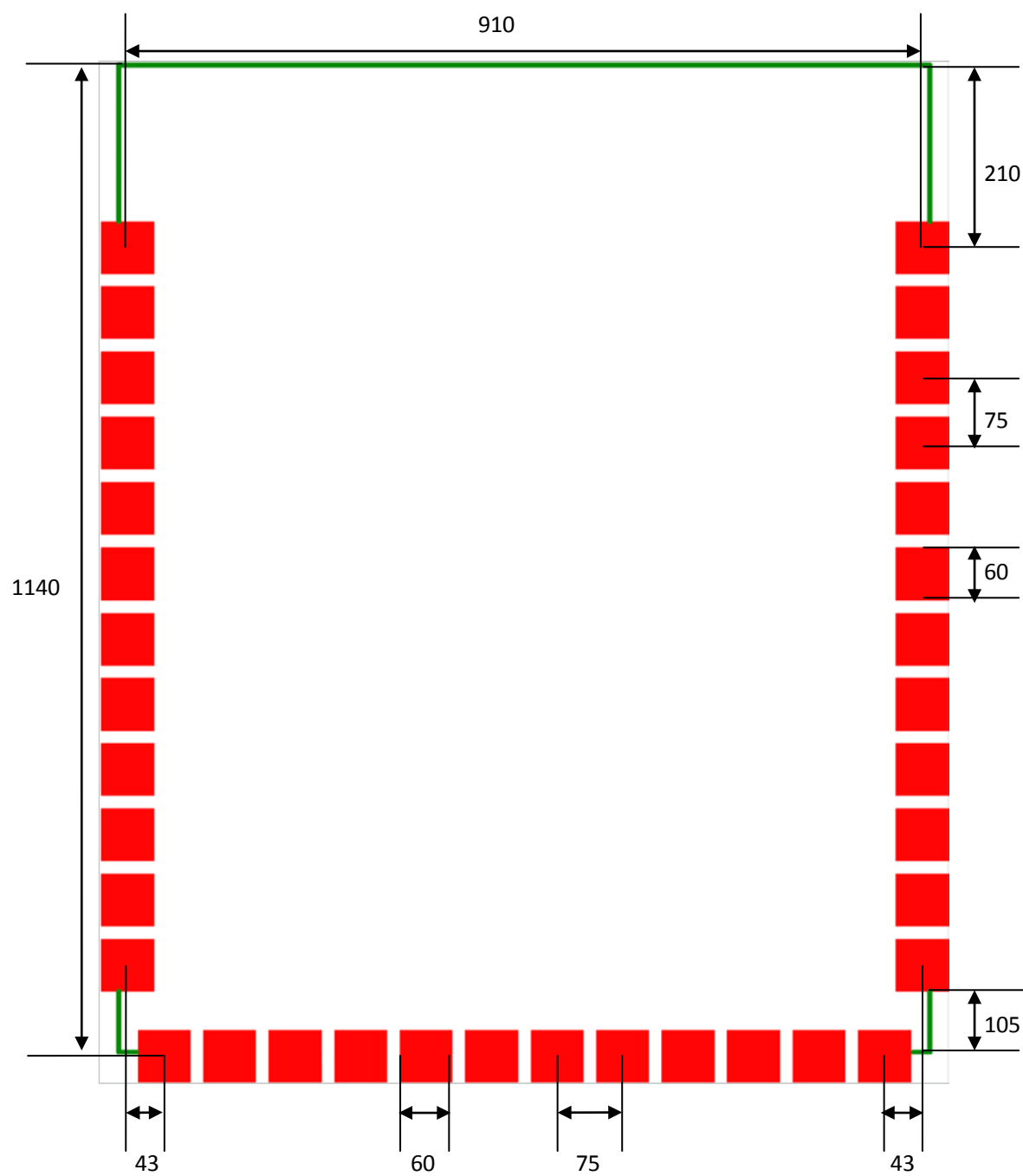
图 4:PCB 引脚焊接(俯视图) (单位 : mil )
