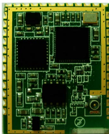
图 1:模块俯视图
