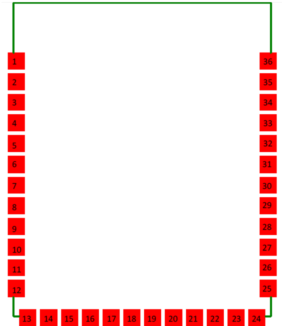
图 7:模块引脚排列图
