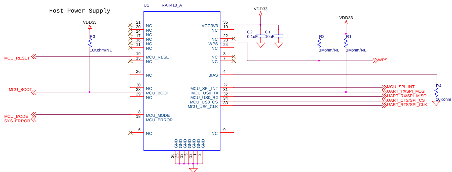
图 5：RAK410 模块外围参考设计图
