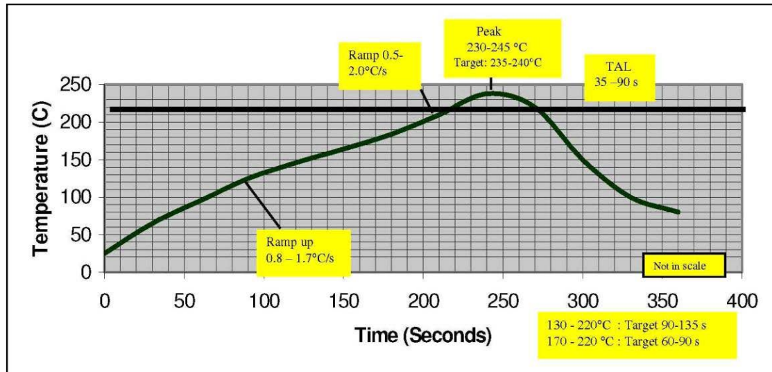
图 6:温度曲线图
