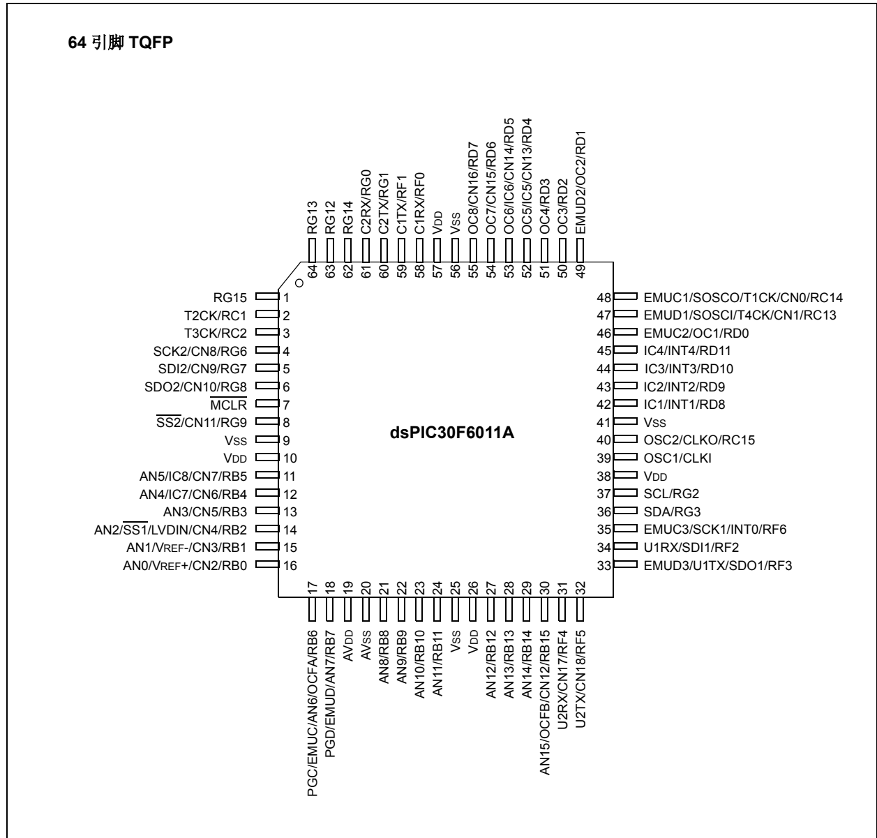
引脚排列图
