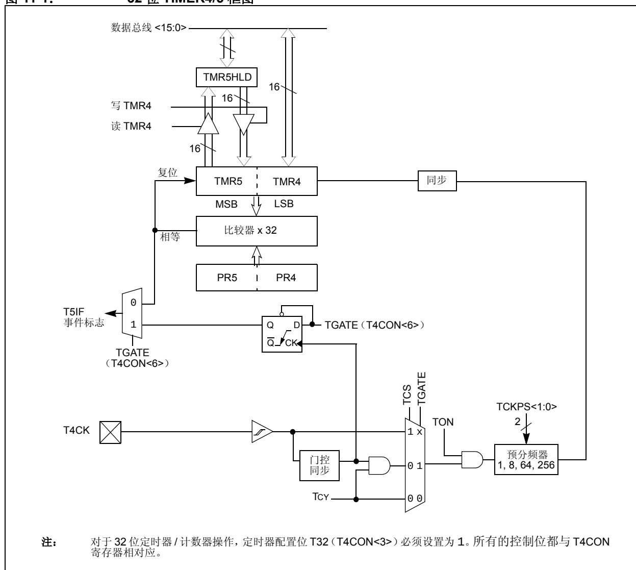
图 11-1: 32 位 TIMER4/5 框图
