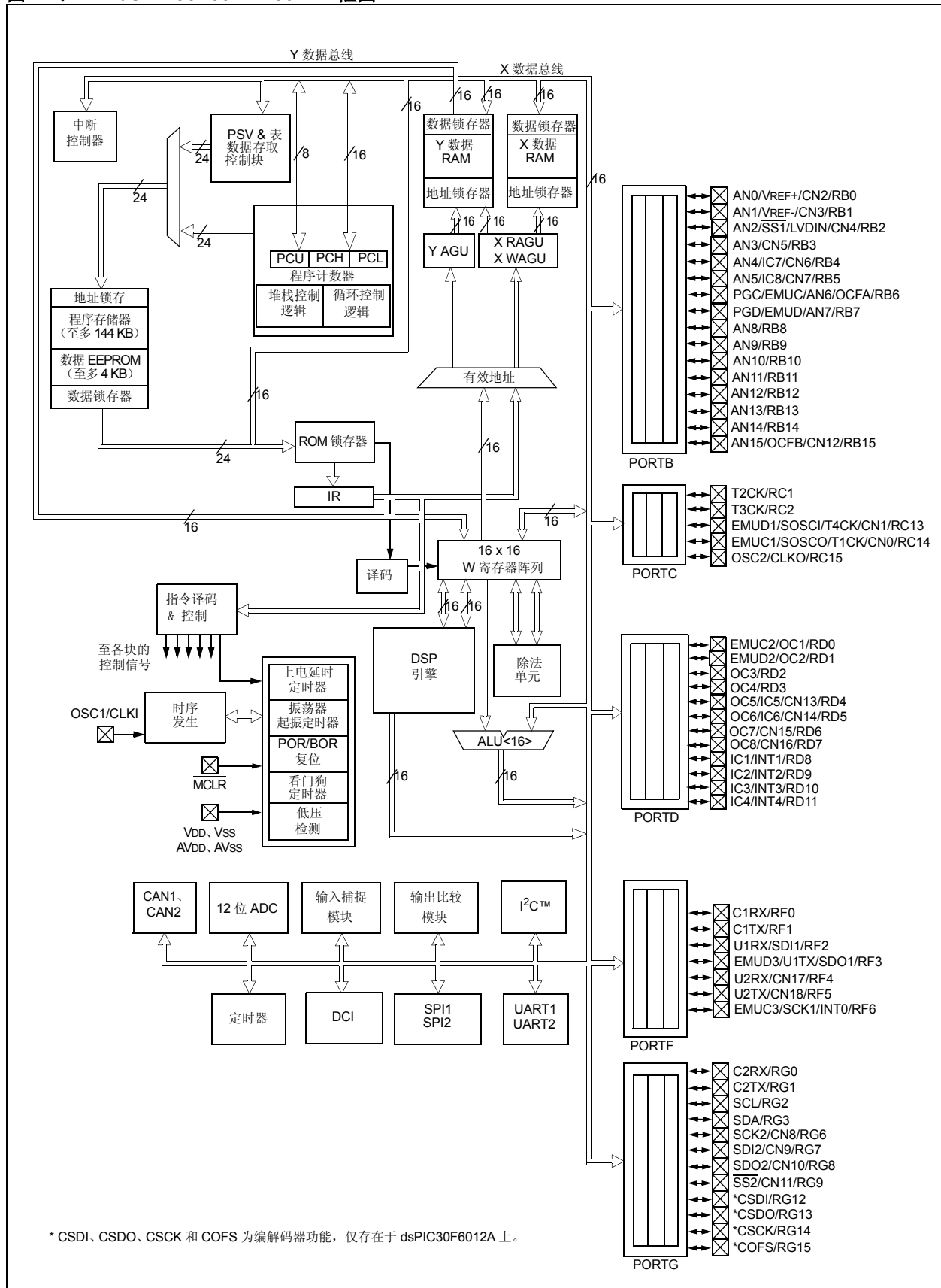
图 1-1: dsPIC30F6011A/6012A 框图
