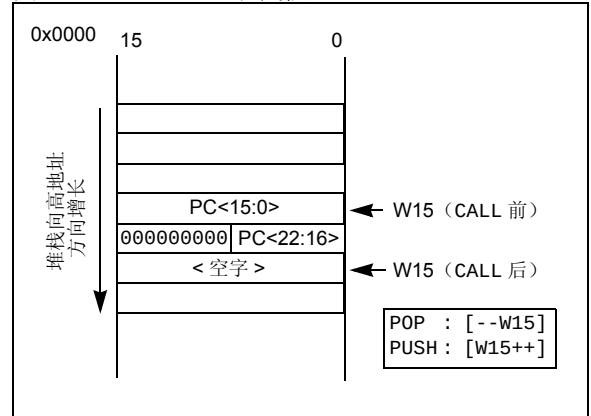
图 3-11: CALL 堆栈帧
