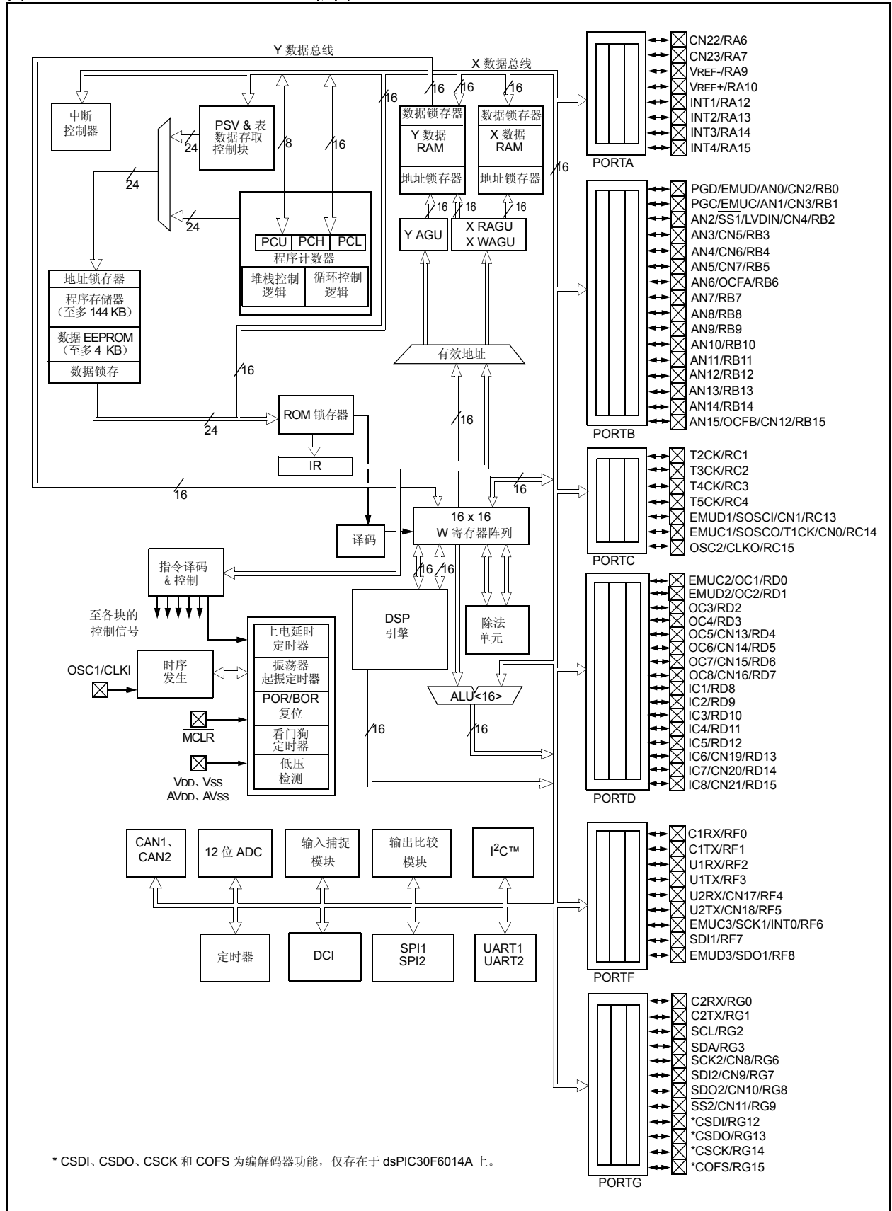
图 1-2: dsPIC30F6013A/6014A 框图
