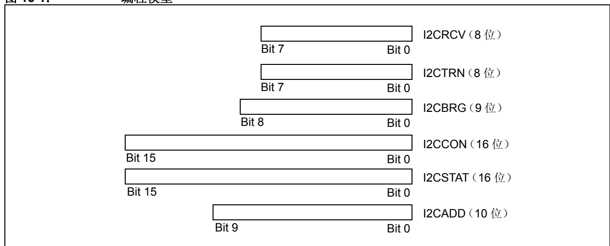
图 15-1: 编程模型
