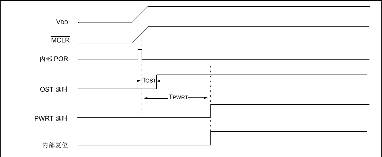
图 20-3: 上电时的延时顺序（MCLR 连接到 VDD）
