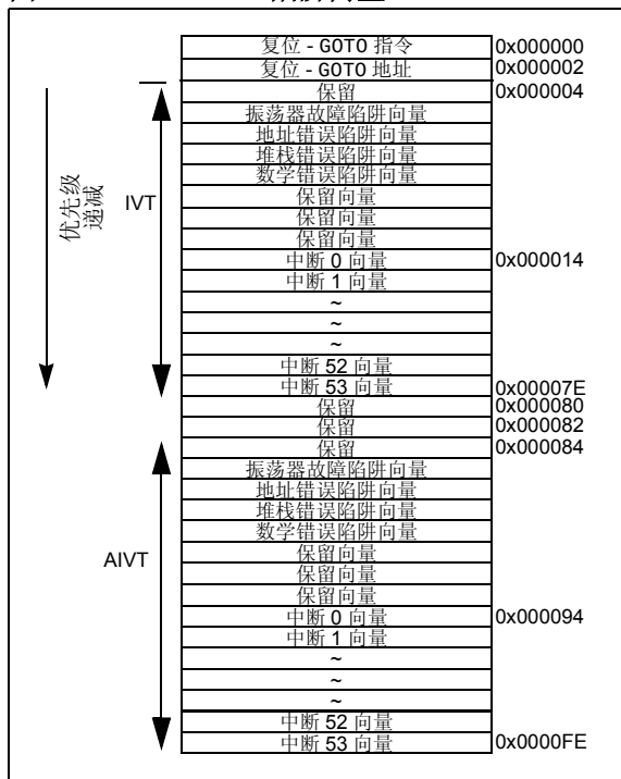
图 5-1: 陷阱向量
