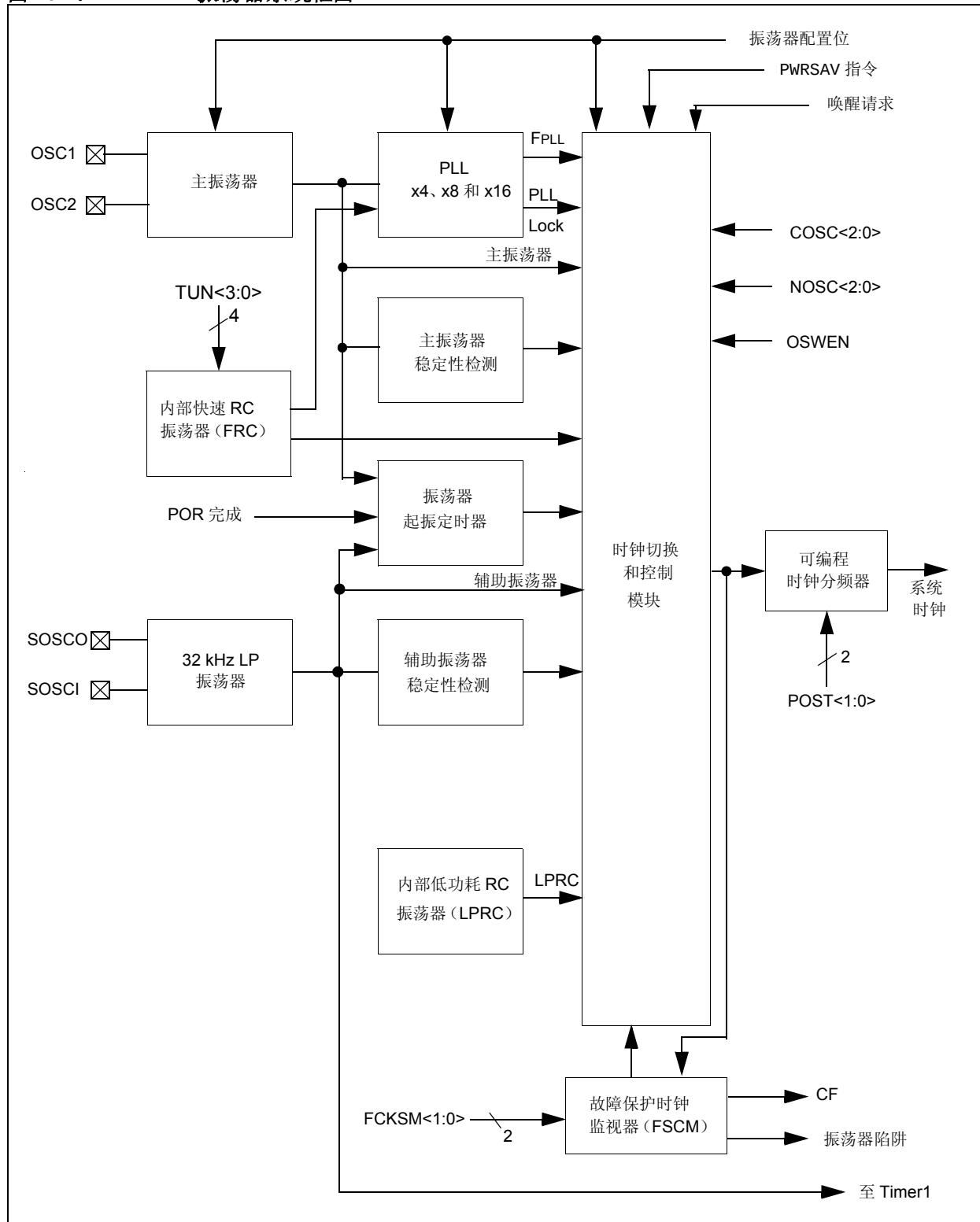
图 20-1: 振荡器系统框图
