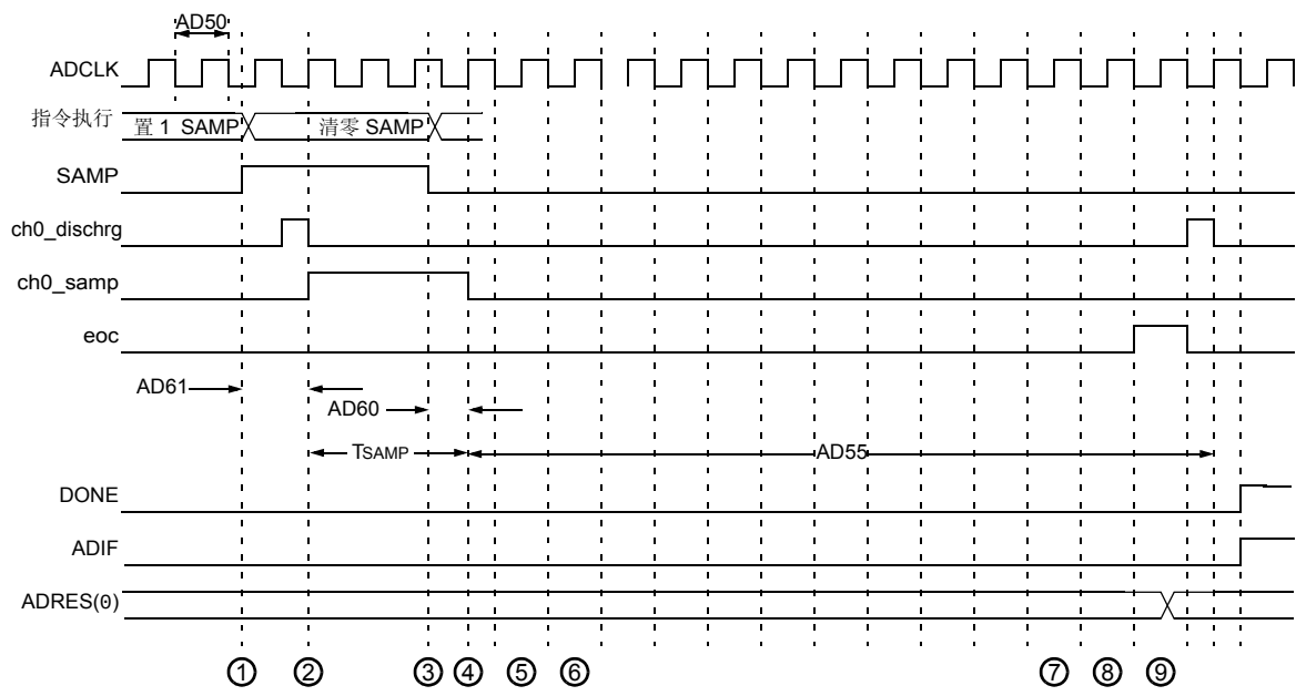
图 23-23: 12 位 ADC 时序特性 (ASAM = 0, SSRC = 000)
