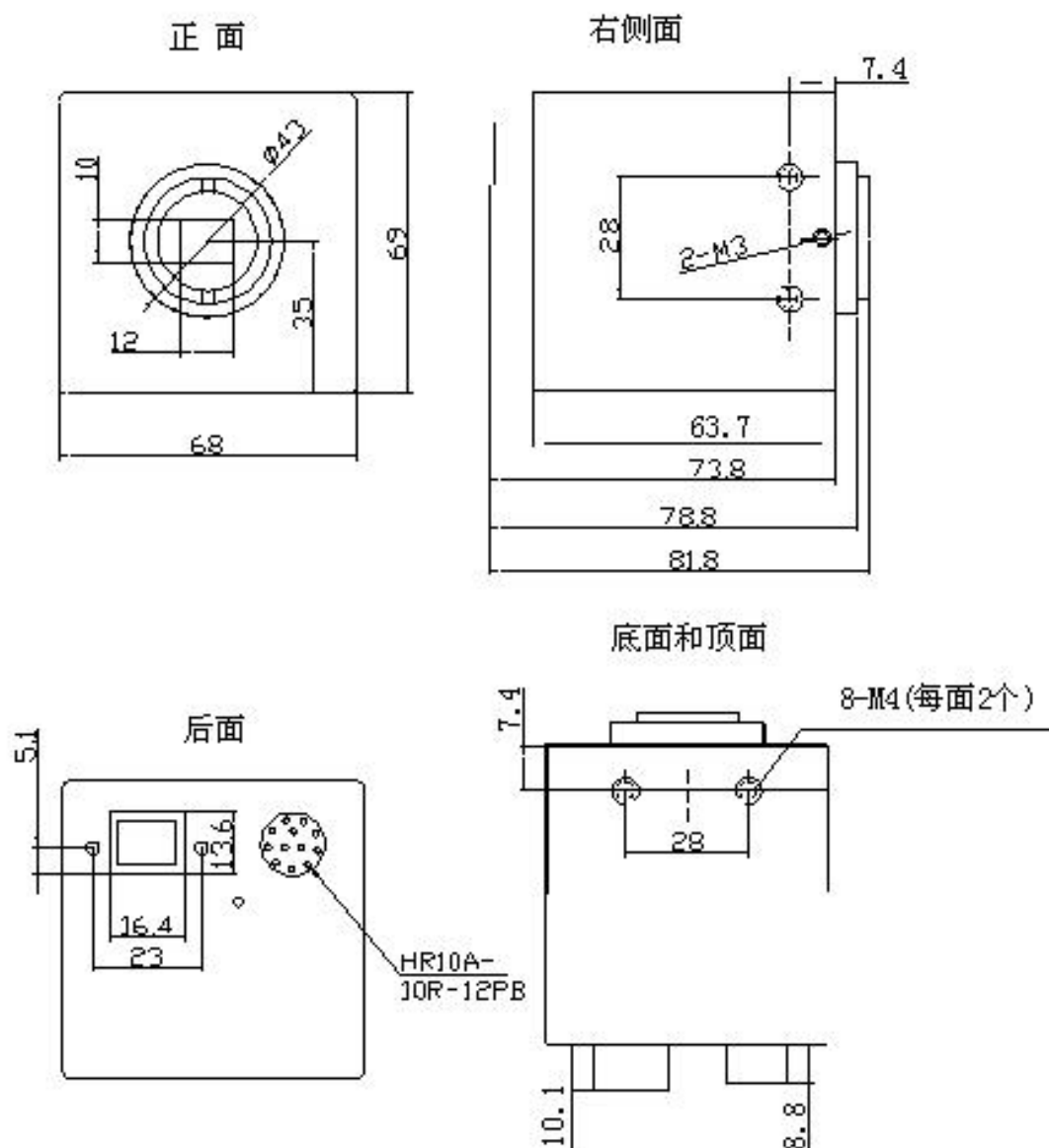
图 2 MVC1800DAM-GE30 的外形尺寸图
