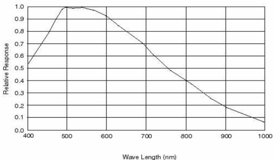
图 1 MVC1800DAM-GE30 的光谱曲线
