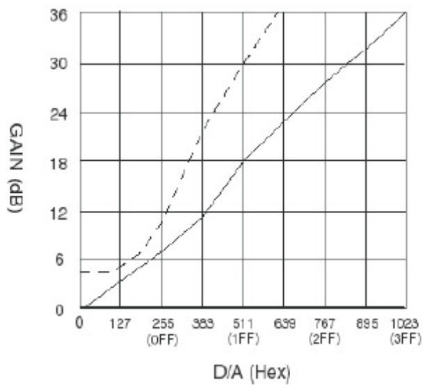
图 4 MVC1800DAM-GE30 增益控制曲线
