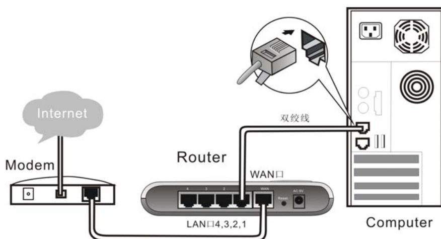
图2-1 线缆连接示意图（DSL/Cable Modem 宽带接入用户）
