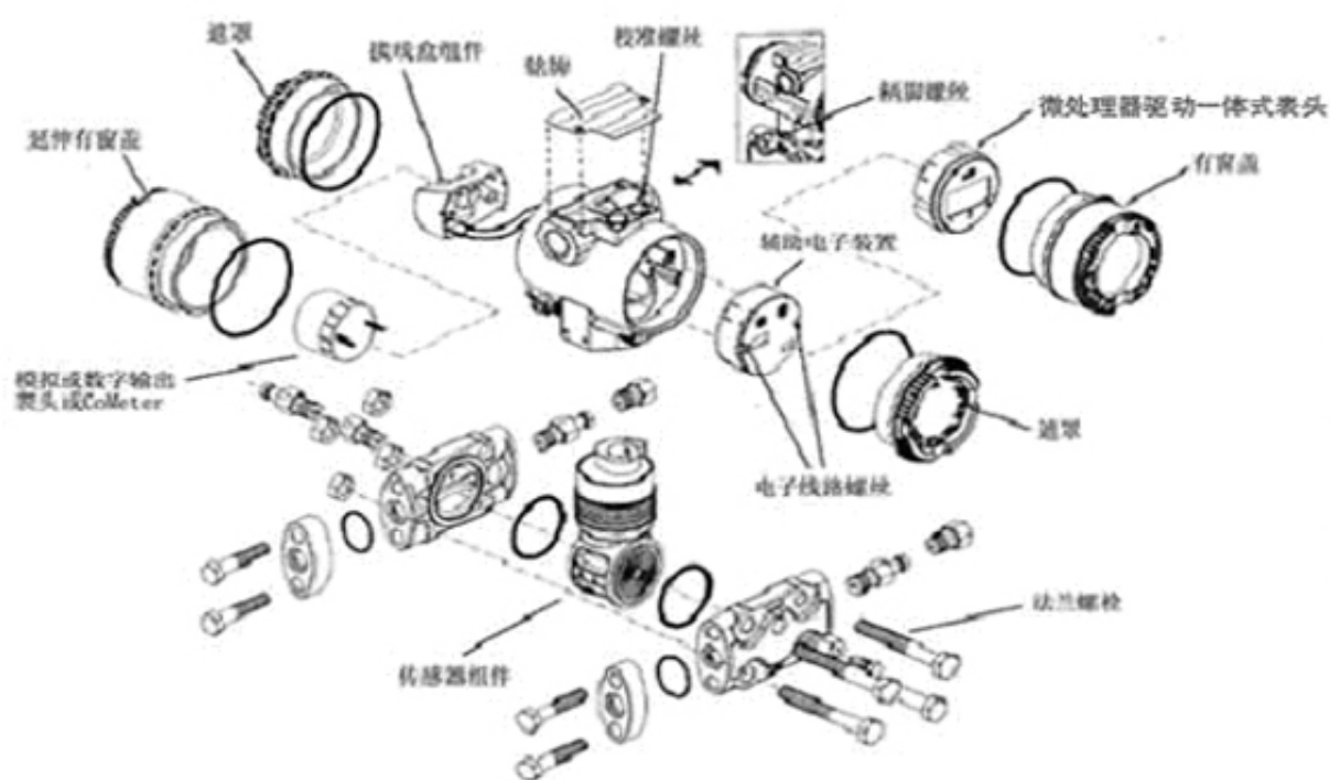
图13a - 264DS/PS/VS型变送器的截面图
