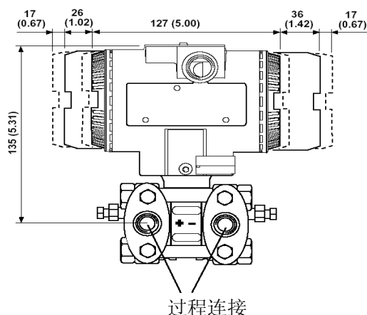
图 6 – 过程连接尺寸图（差压变送器）
