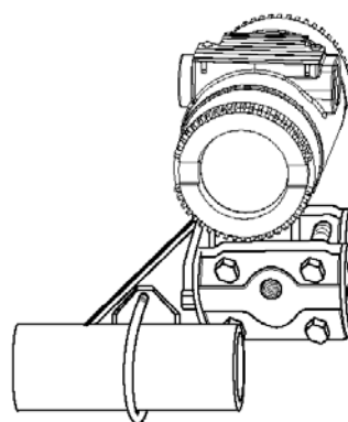
图 5-安装在 2 英寸水平管上
