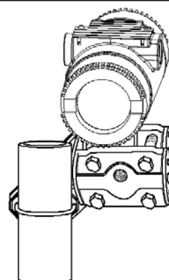
图 4-安装在 2 英寸垂直管上
