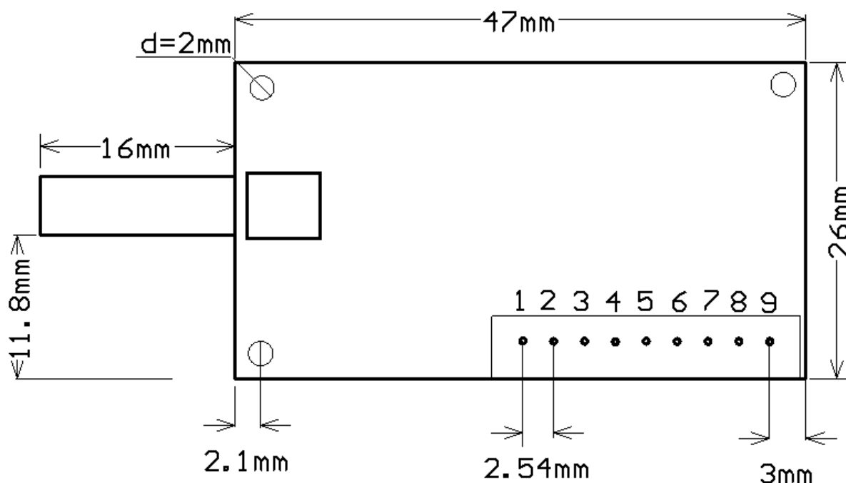
KYL-1020U 接口示意图
