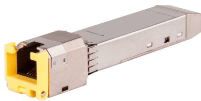
图11-5 千兆 SFP 电口光模块外观示意图
