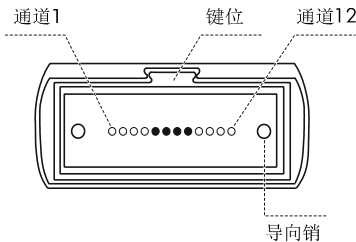
图1-4 12 芯光纤的 MPO 连接器俯视图
