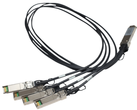
图2-4 QSFP28 to SFP28 电缆示意图
