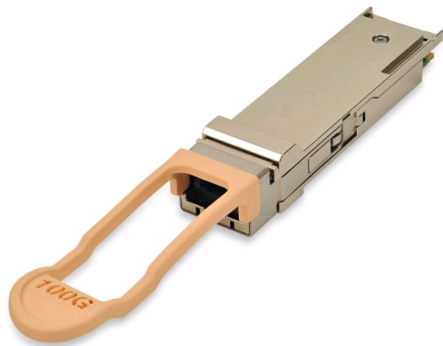
图2-1 QSFP28 光模块（MPO 接口）外观示意图
