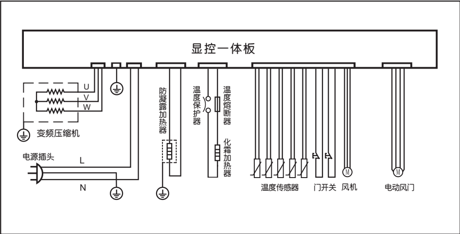
电路图
