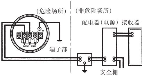
图 5.4.1b 变送器与配电器的连接
