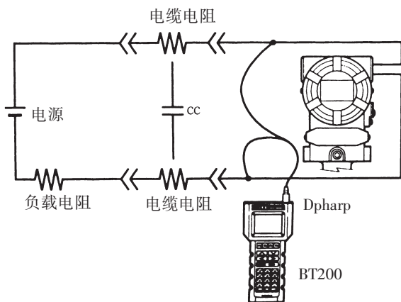
图 7.1.2 回路
