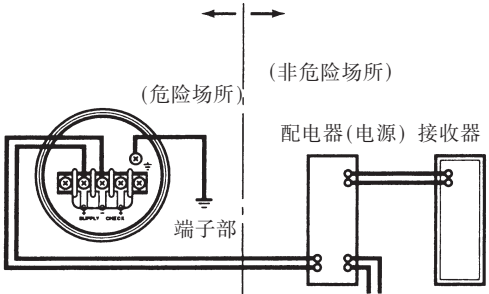
图 5.4.1a 变送器与配电器的连接
