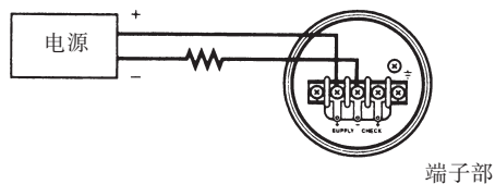
图 5.3.1 电源连接
