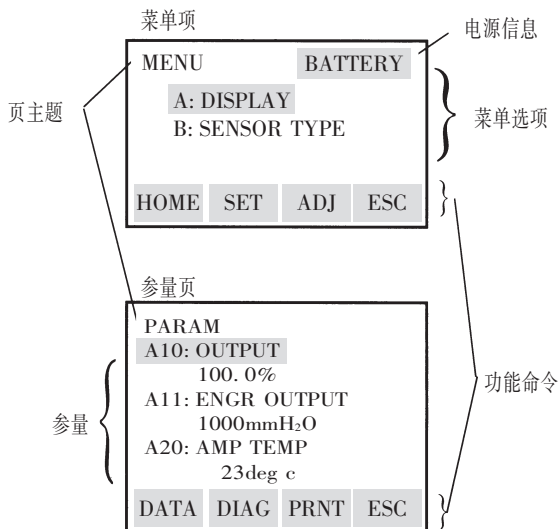
图 7.2.1 BT200 键面图
