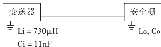
图 2.5 安全栅连接图
