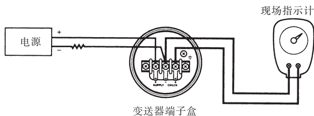
图 5.3.2 外接指示计连接
