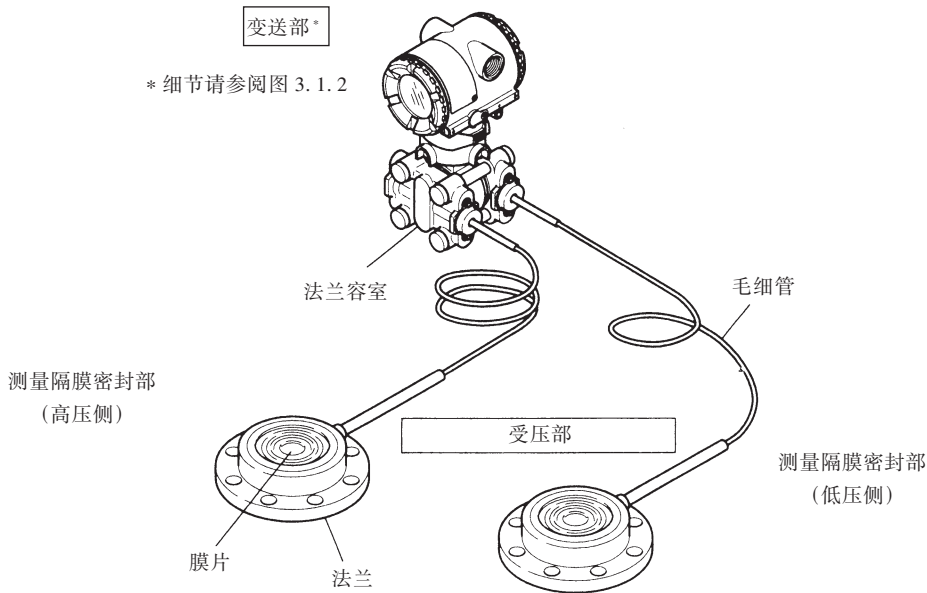
图 3.1.1 各部件名称(EJA118W)
