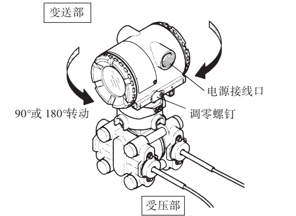
图 4.5.1 变送部的转动
