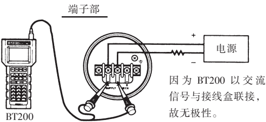
图 5.3.3 BT200 的连接
