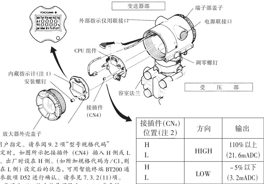
图 3.1.1 各部件名称(EJA118W)
