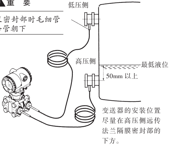
图 4.2 液罐安装实例
