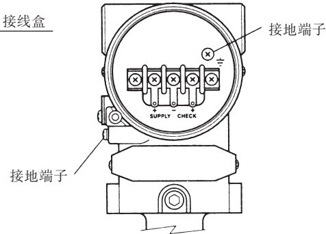
图 5.5 接地端子
