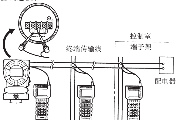
图 7.1.1 BT200 的连接
