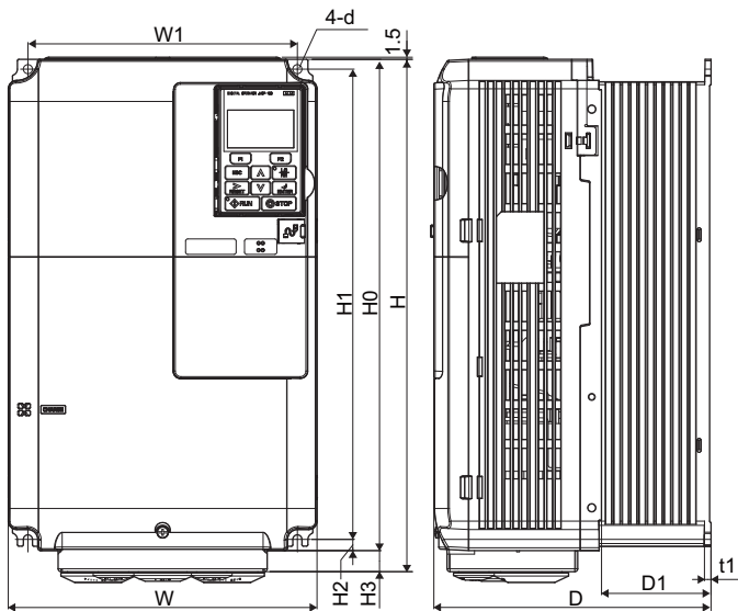
外形图 2
