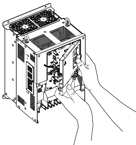
图 22 前外罩的拆卸 (2A0085 ~ 2A0415、4A0045 ~ 4A1090)
