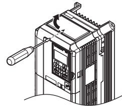
图 24 上部保护罩的拆卸
