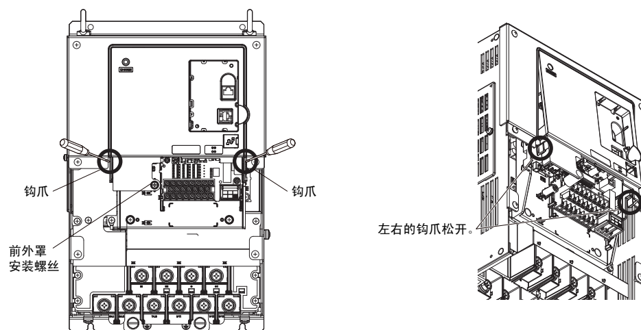
图 21 前外罩的拆卸 (2A0085 ~ 2A0415、4A0045 ~ 4A1090)
