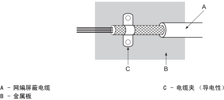
图 120 电缆的接地方法
