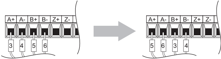
图 116 A 相和 B 相信号线的调换
