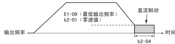
图 60 无 PG V/f 控制、带 PG V/f 控制、无 PG 矢量控制时的停止时直流制动动作
