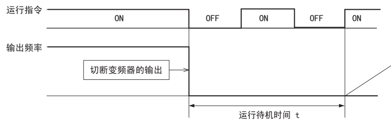
图 58 带定时的自由运行停止
