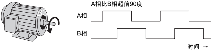
图 115 A 相、B 相信号相位关系图
