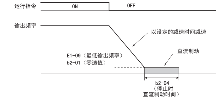
图 52 减速停止（无 PG V/f 控制、带 PG V/f 控制、无 PG 矢量控制模式）
