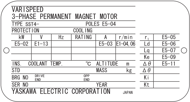
图 80 电机铭牌（例）
