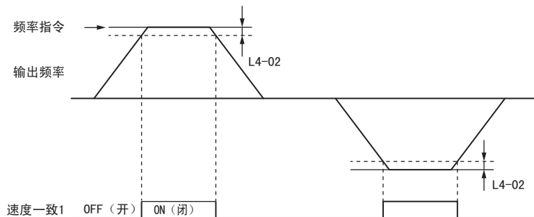
图 69 速度一致 1 的时序图
