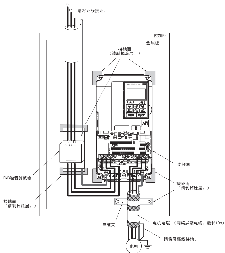
图 121 EMC 噪音滤波器和变频器的安装方法 (三相 200V/400V 级)
