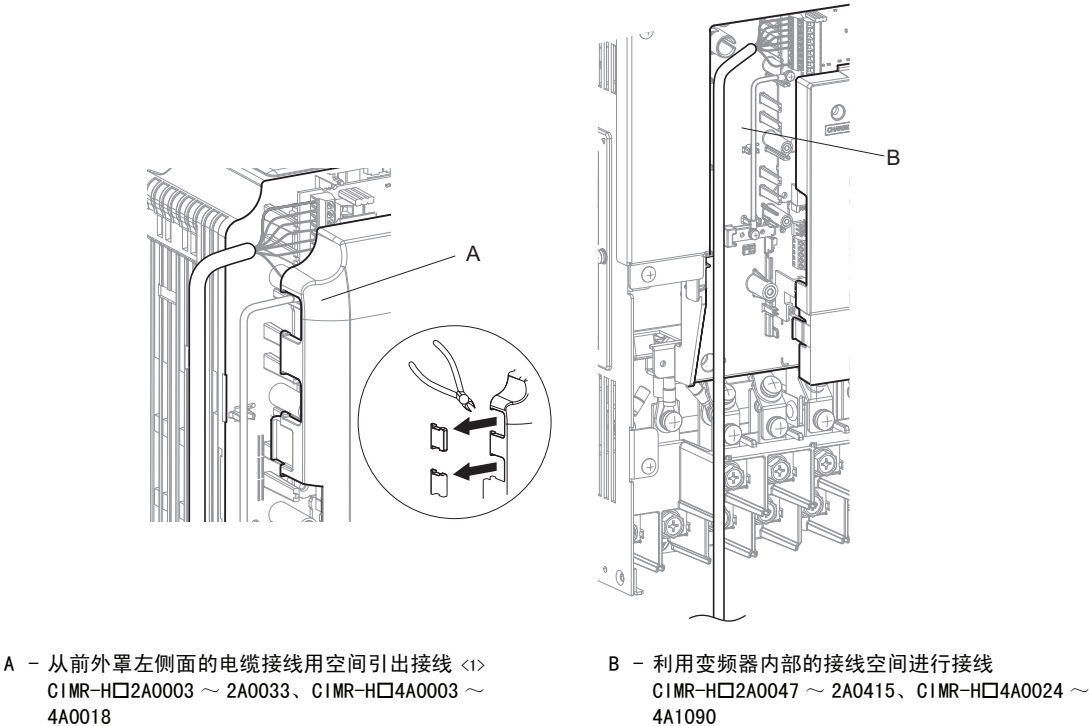
图 113 电缆的接线方法
