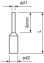
图 32 棒端子的外形尺寸图
