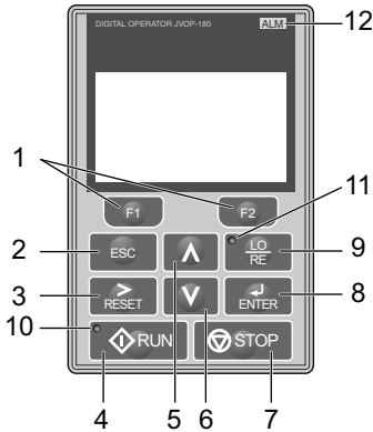
图 44 操作器各部分的名称与功能
