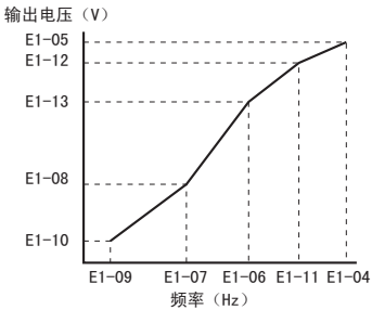
图 66 V/f 曲线图
