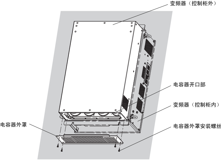
图 125 电容器外罩的安装
