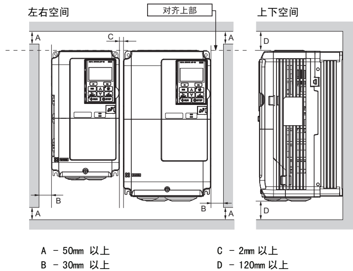
图 6 变频器的安装空间（并列安装）
