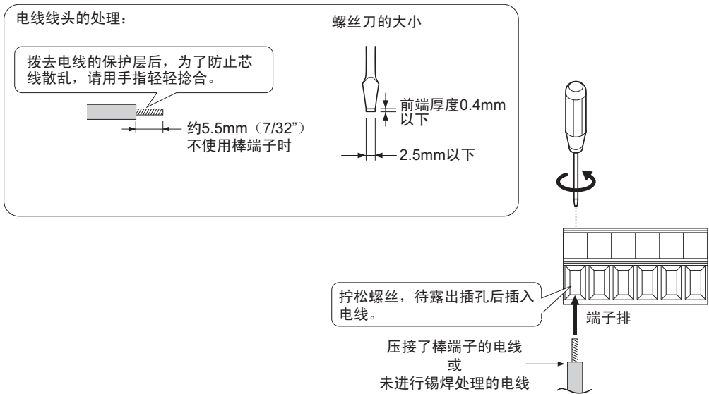
图 106 向端子排的接线
