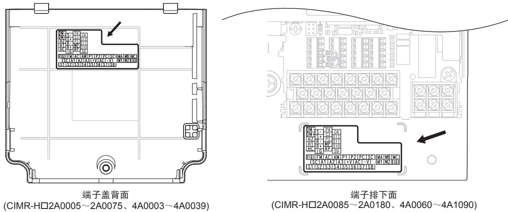
图 31 端子排的排列标示
