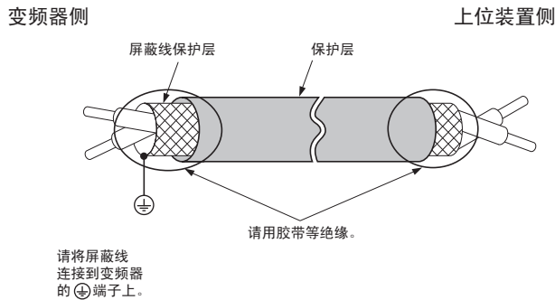
图 35 屏蔽线的线头处理
