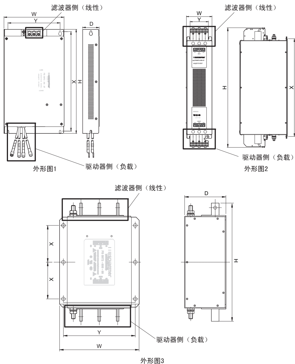
图 122 EMC 噪音滤波器的外形尺寸
