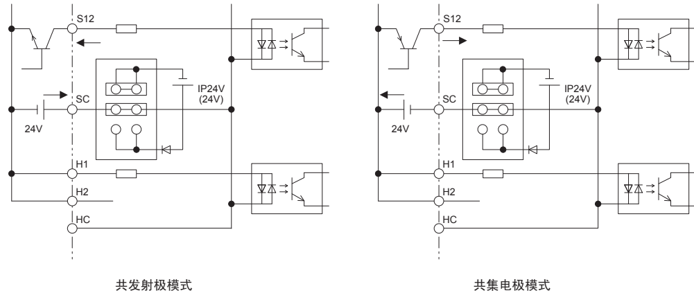
图 39 不使用安全输入时的接线示例
