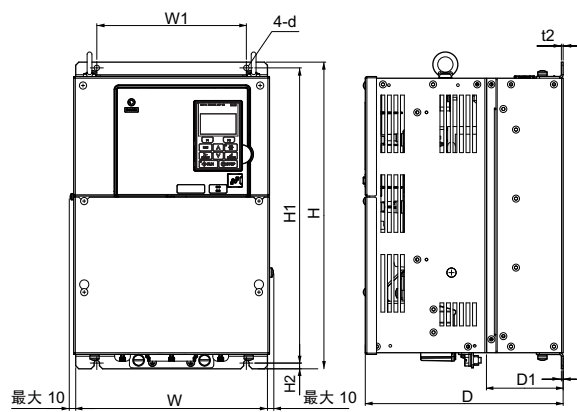
外形图 1
