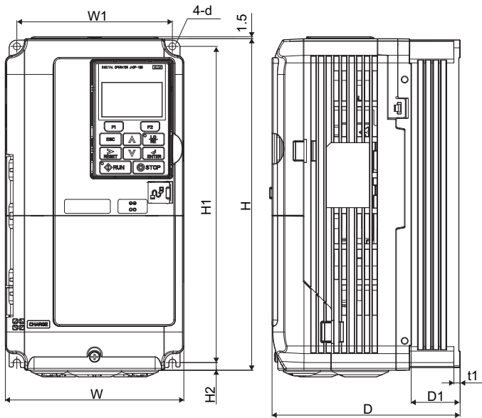
外形图 1
