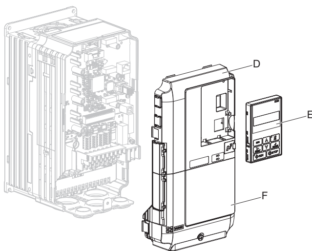
图 102 操作器、前外罩的拆卸
