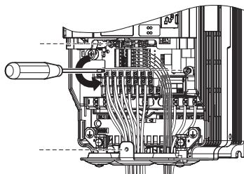
图 97 变频器的更换（拧松固定螺丝）
