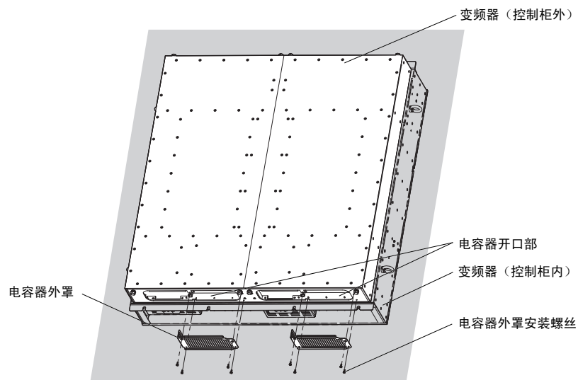
图 126 电容器外罩的安装（4A0810、4A1090）
