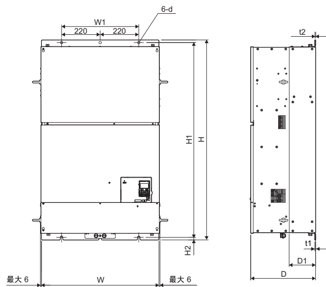
外形图 3
