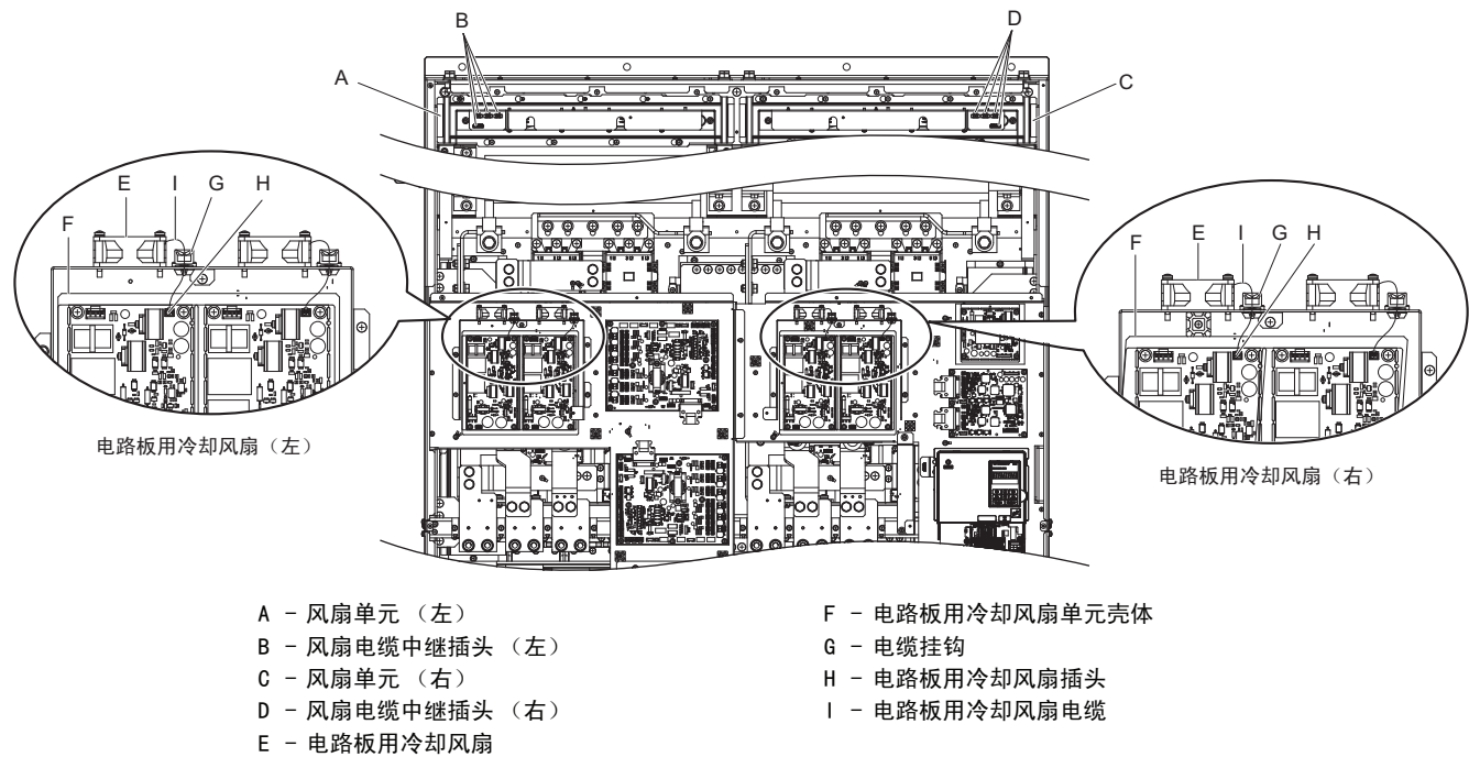
图 82 各部分的名称：4A0810、4A1090
