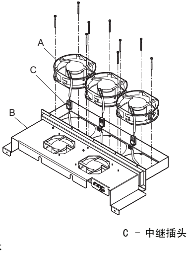
图 85 冷却风扇的更换：4A0810、4A1090
