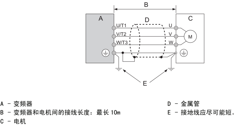
图 119 安装方法
