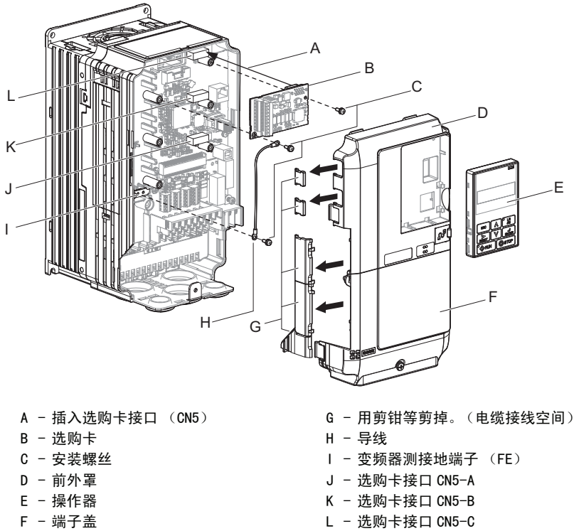
图 101 变频器和选购卡
