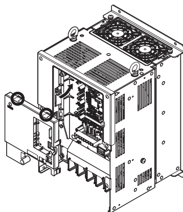
图 23 前外罩的安装 (2A0085 ~ 2A0415、4A0045 ~ 4A1090)
