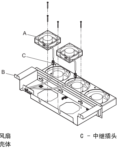
图 87 内气搅动风扇的更换：4A0810、4A1090
