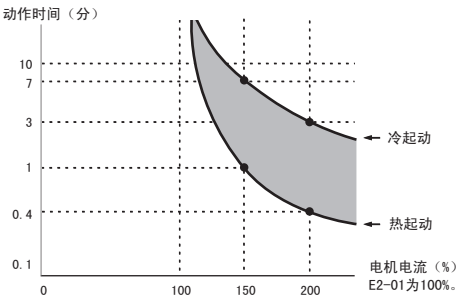
图 124 由输出频率和负载决定的电机过载保护时间
