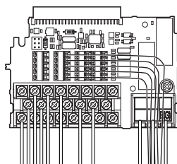
图 99 变频器的更换 (已拆下的拆装式端子排)
