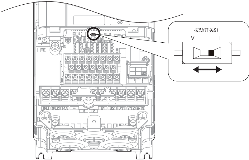
图 42 拨动开关 S1
