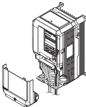
图 96 变频器的更换（端子外罩的拆卸）
