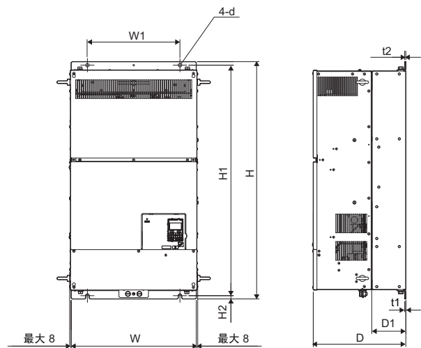
外形图 2
