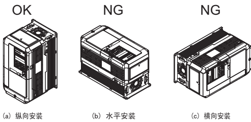
图 4 安装方向
