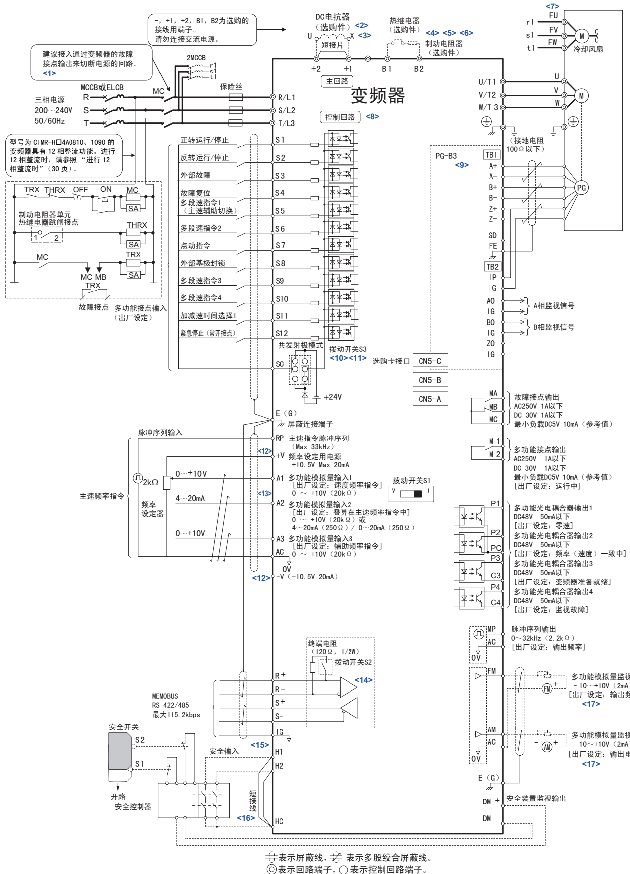
图 8 变频器的标准接线图 (例: CIMR-H□2A0033)
