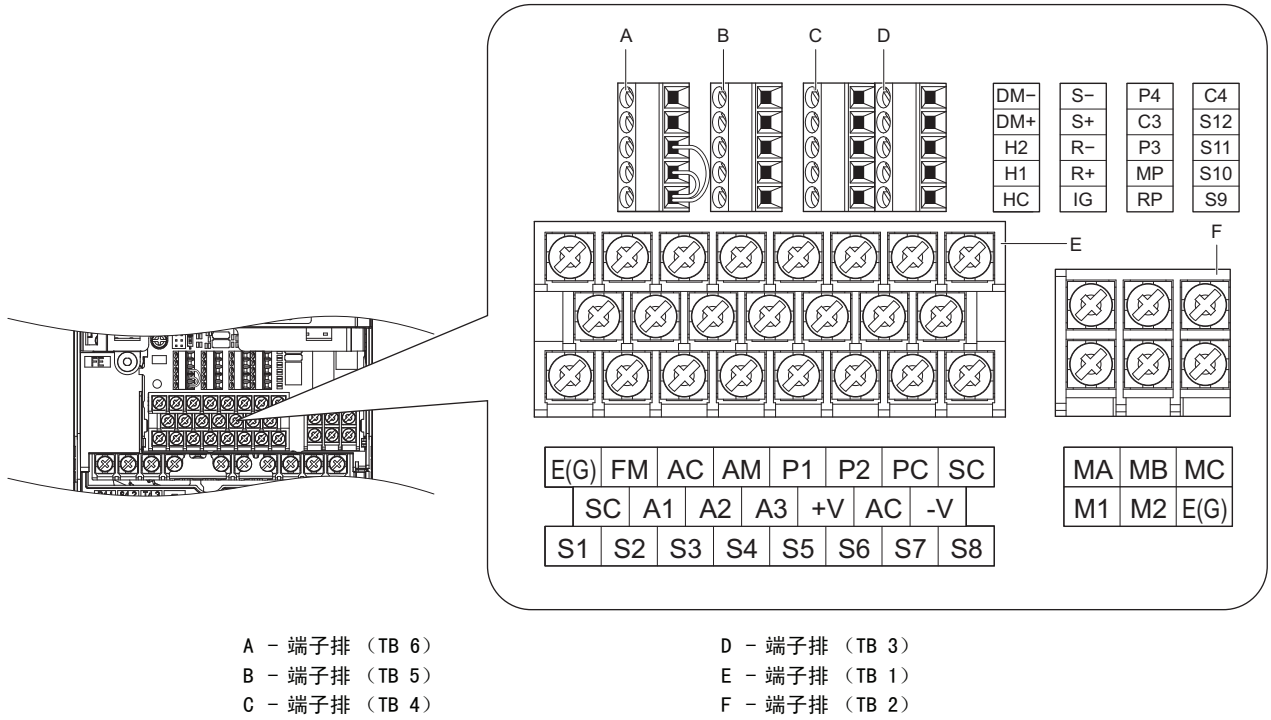
图 30 带参数备份功能的拆装式端子排的排列 (CIMR-HB□□□□□□□□)
