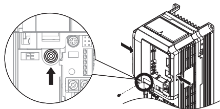
图 20 前外罩的拆卸（2A0005 ~ 2A0075、4A0003 ~ 4A0039）
