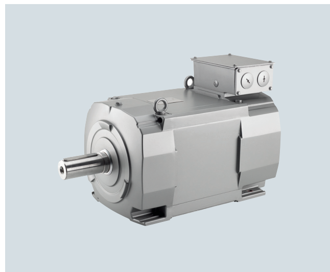
1PH8 电机，水冷，轴高 180-280
