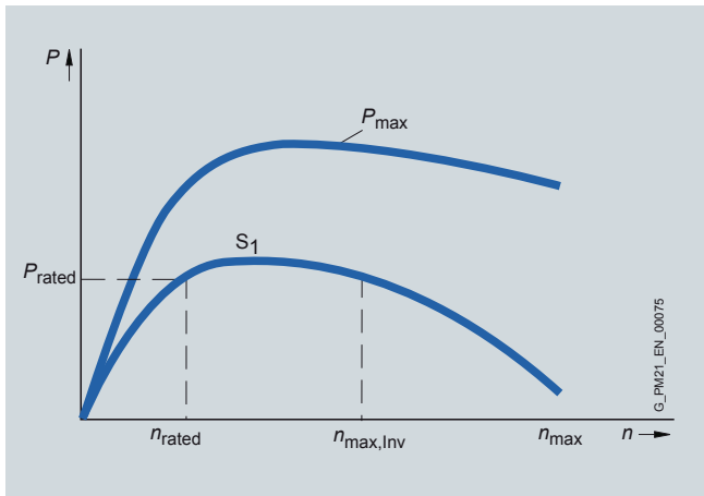
1PH8 同步电机典型速度 / 功率特性
