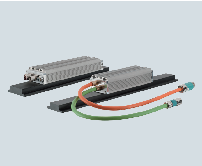
1FN6 直线电机，左侧：集成两个插座，分别用做驱动和信号线缆连接；右侧：带有永久链接的驱动和信号电缆
