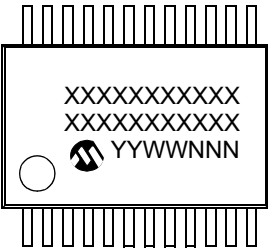
24 引脚 SSOP
