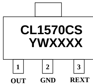
SOT-89-3L
