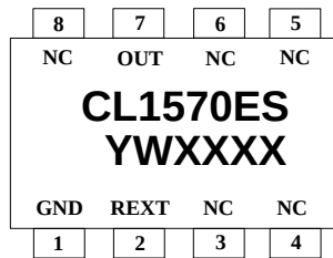
ESOP8
