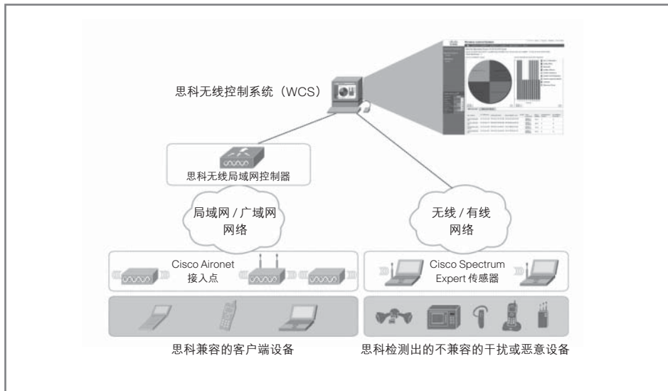
图 1 思科频谱智能解决方案的拓扑图
