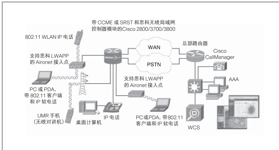
图2 拥有安全数据、语音、交换和无线功能的有线和无线融合型分支机构
