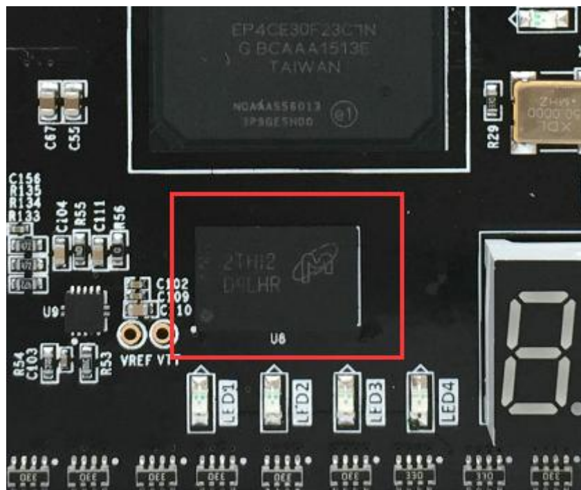
图 7.2 为 DDR2 DRAM 实物图
