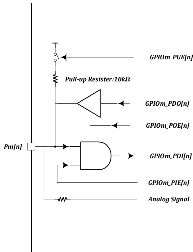
图 15-1 GPIO 功能框图
