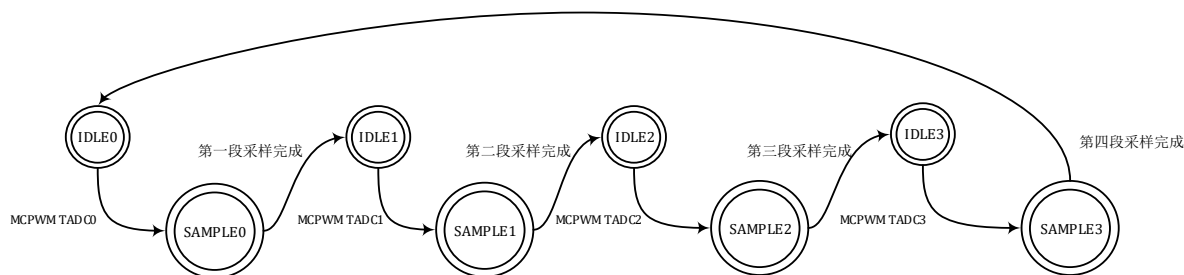
图 12-5 ADC 四段采样状态转移图
