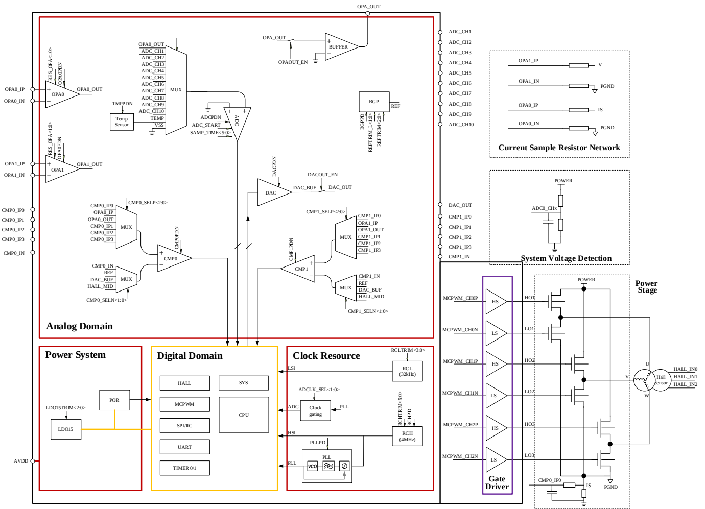
图 5-1 模拟电路功能框图
