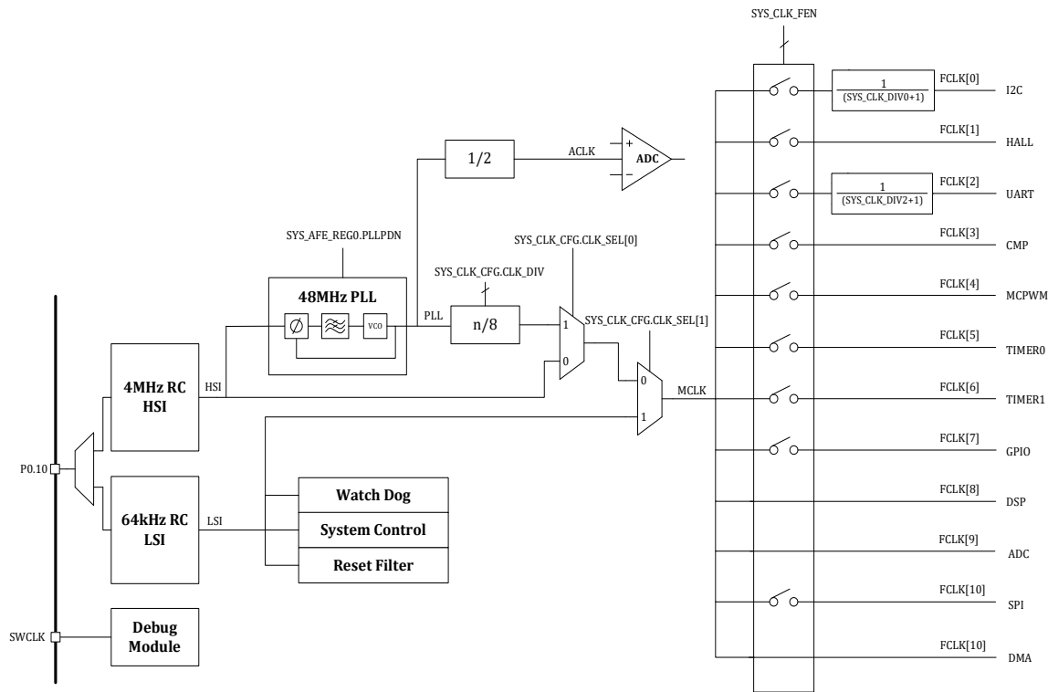
图 6-1 时钟架构
