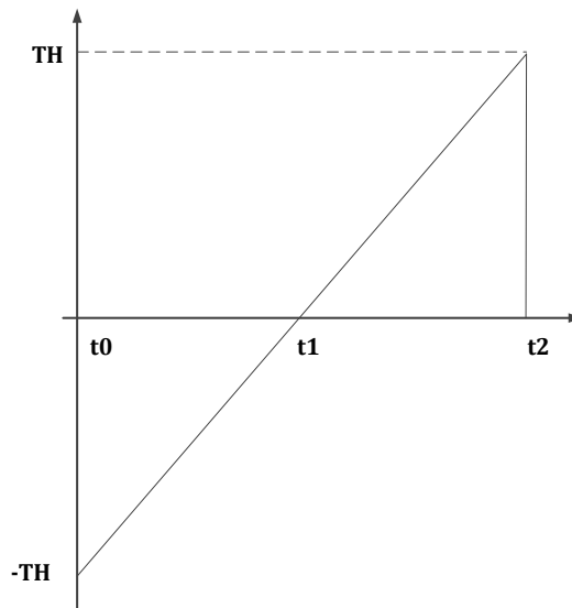
图 14-2 Base Counter t_0/t_1 时序
