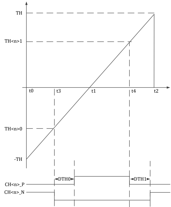
图 14-7 MCPWM 时序 TH_{<n>0} 和 TH_{<n>1} -中心对齐模式
