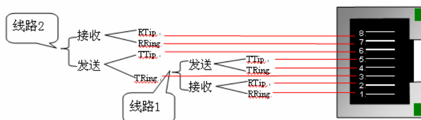
图 2-6 复用 RJ48C 接口的引线
