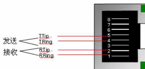
图 2-5 普通 RJ48C 接口的引线
