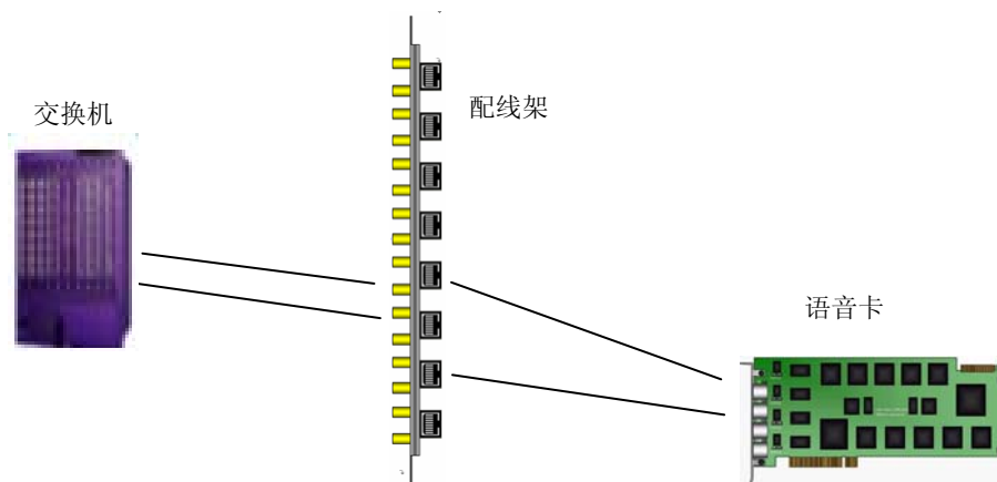
图 2-1 接线示意图
