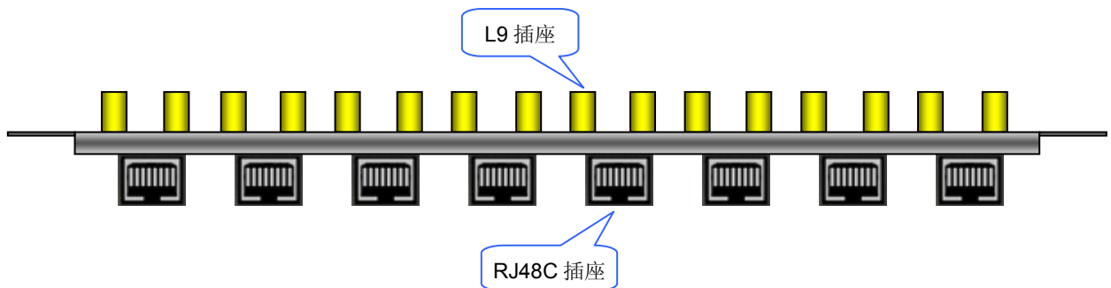
图 2-4 SHD-240A-JB/L9 平视图
