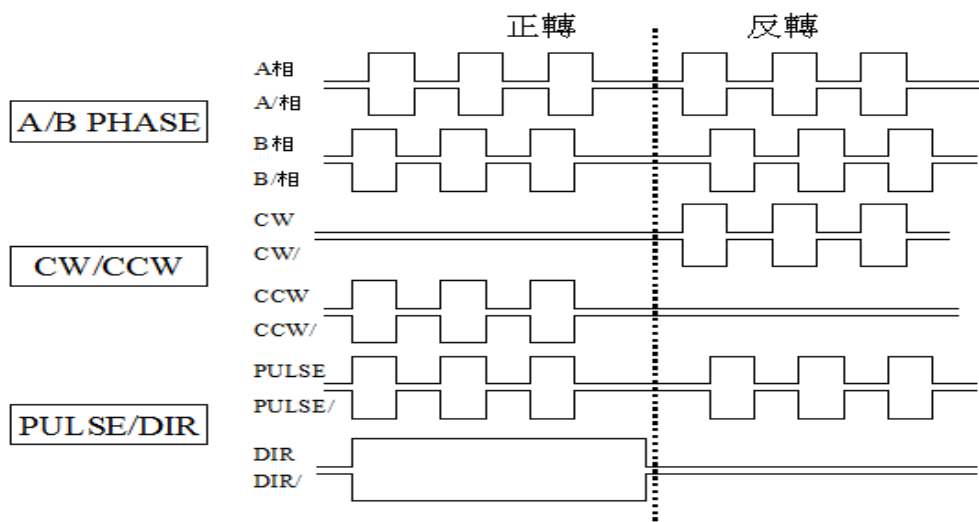
图表 2.2-4 输出脉冲格式示意图
