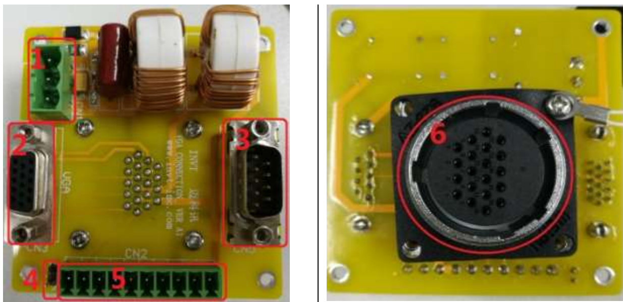
图表 4.3-1 滤波板
