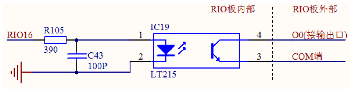
图表 4.5-2 ARIO 输出电路
