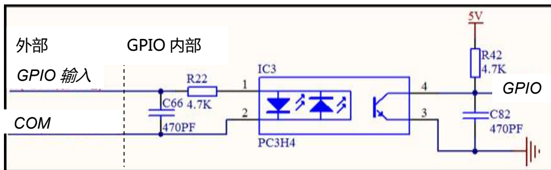
图表 4.4-3 GPIO 输入电路
