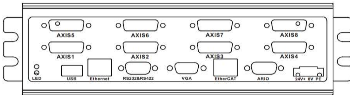
图表 4.2-1 控制器接口定义图 ( 1 )
