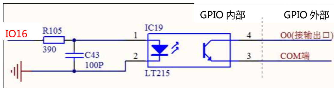
图表 4.4-2 GPIO 输出电路
