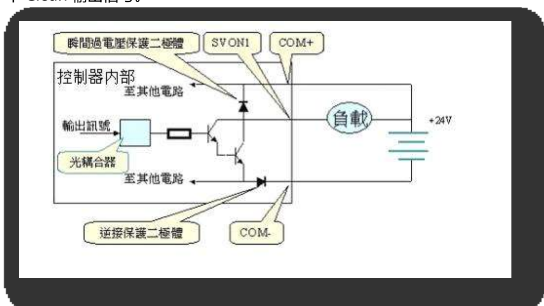
图表 4.4-5 LIO 输出电路
