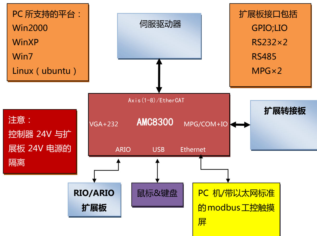
图 2.1-3 A+PC 控制模式结构图
