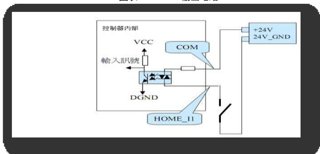
图表 4.4-6 LIO 输入电路
