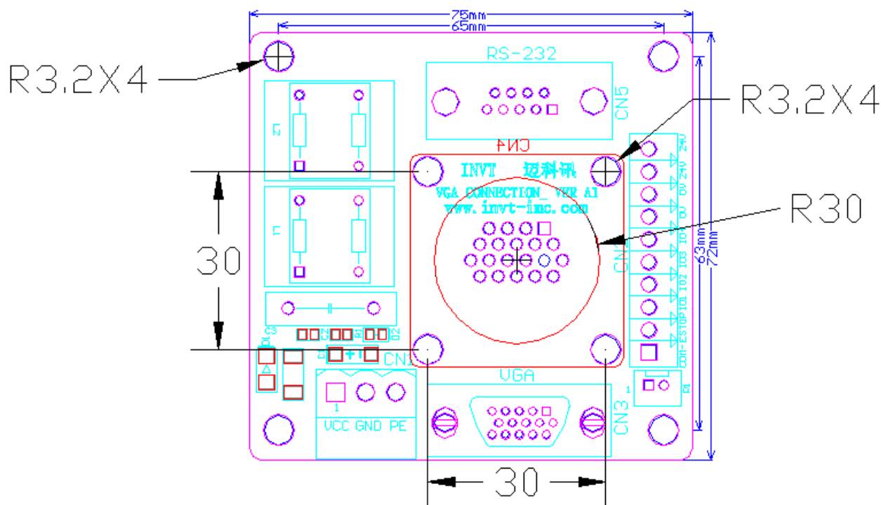
图表 4.3-2 滤波板尺寸图
