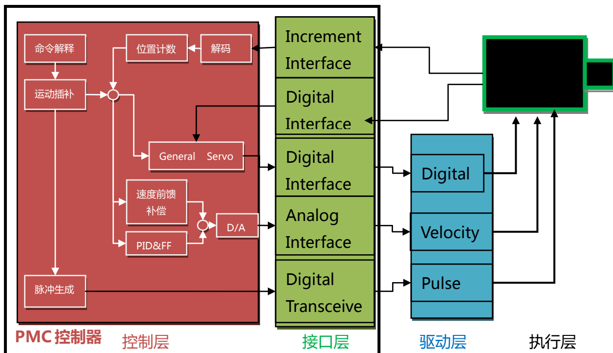
图表 2.2-1 控制模块图
