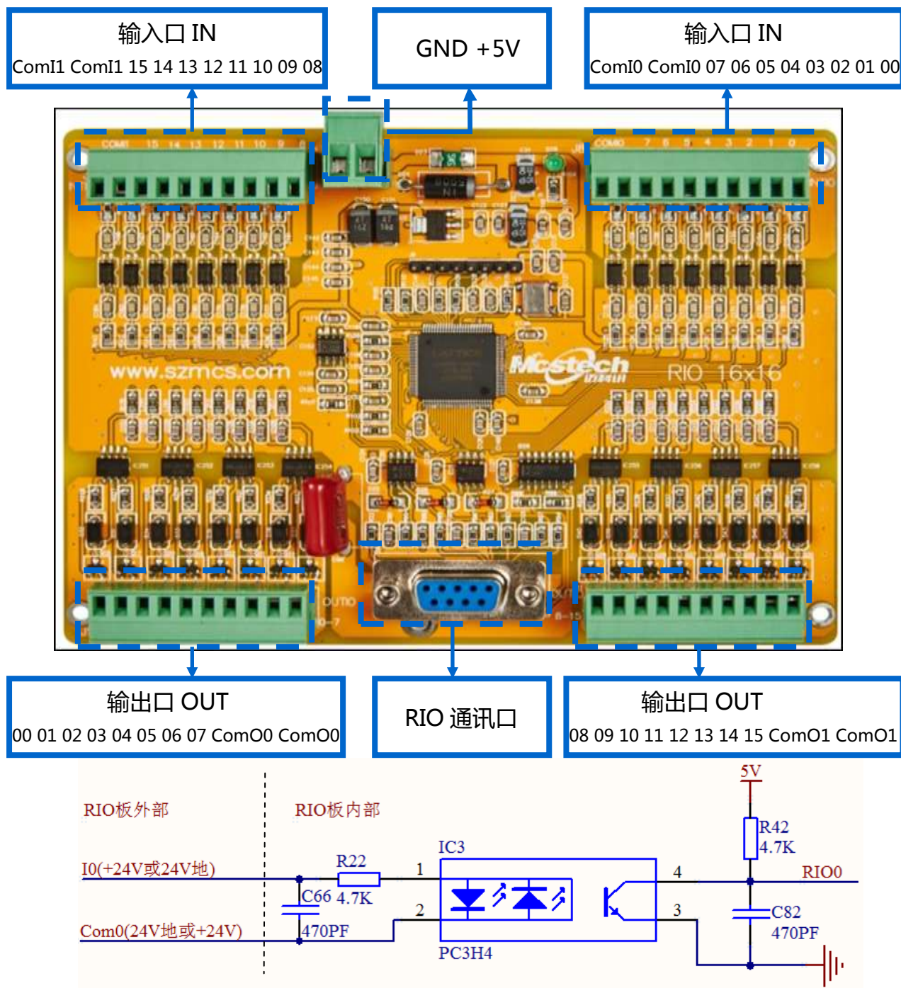
图表 4.5-1 ARIO 输入电路
