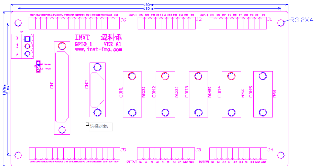
图表 4.4-4 转接板尺寸图
