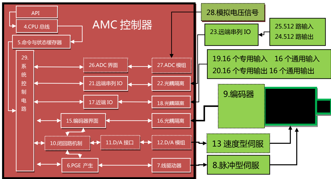
图表 2.2-3 控制框图
