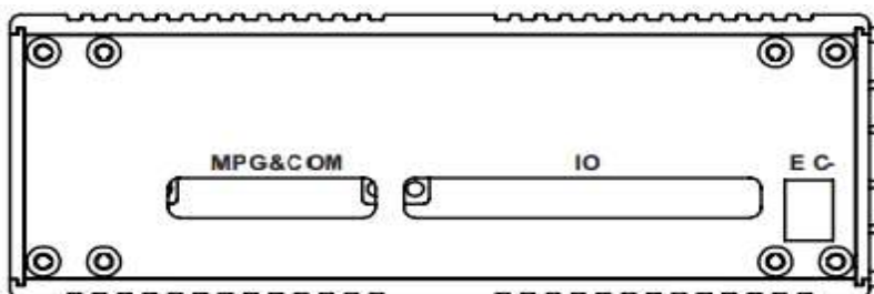
图表 4.2-2 控制器接口定义图 ( 2 )
