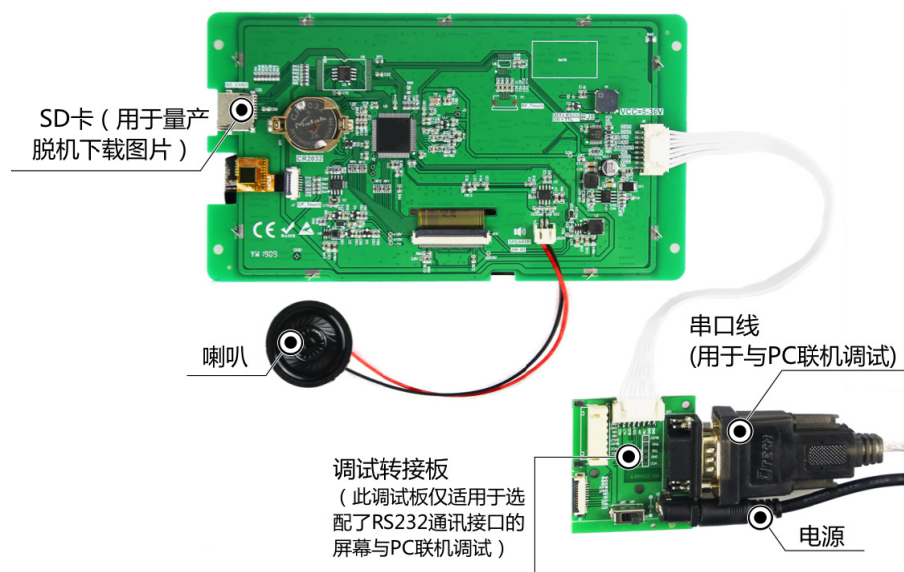
图 1-5 调试工具图
