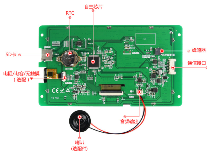
图 1-4 硬件配置图
