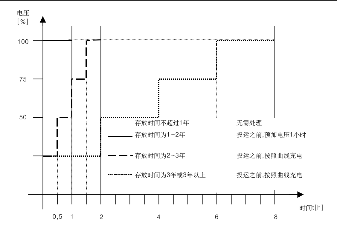
图 2-1 充电
