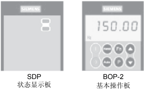
图 3-3 MICROMASTER 430 变频器的操作面板
