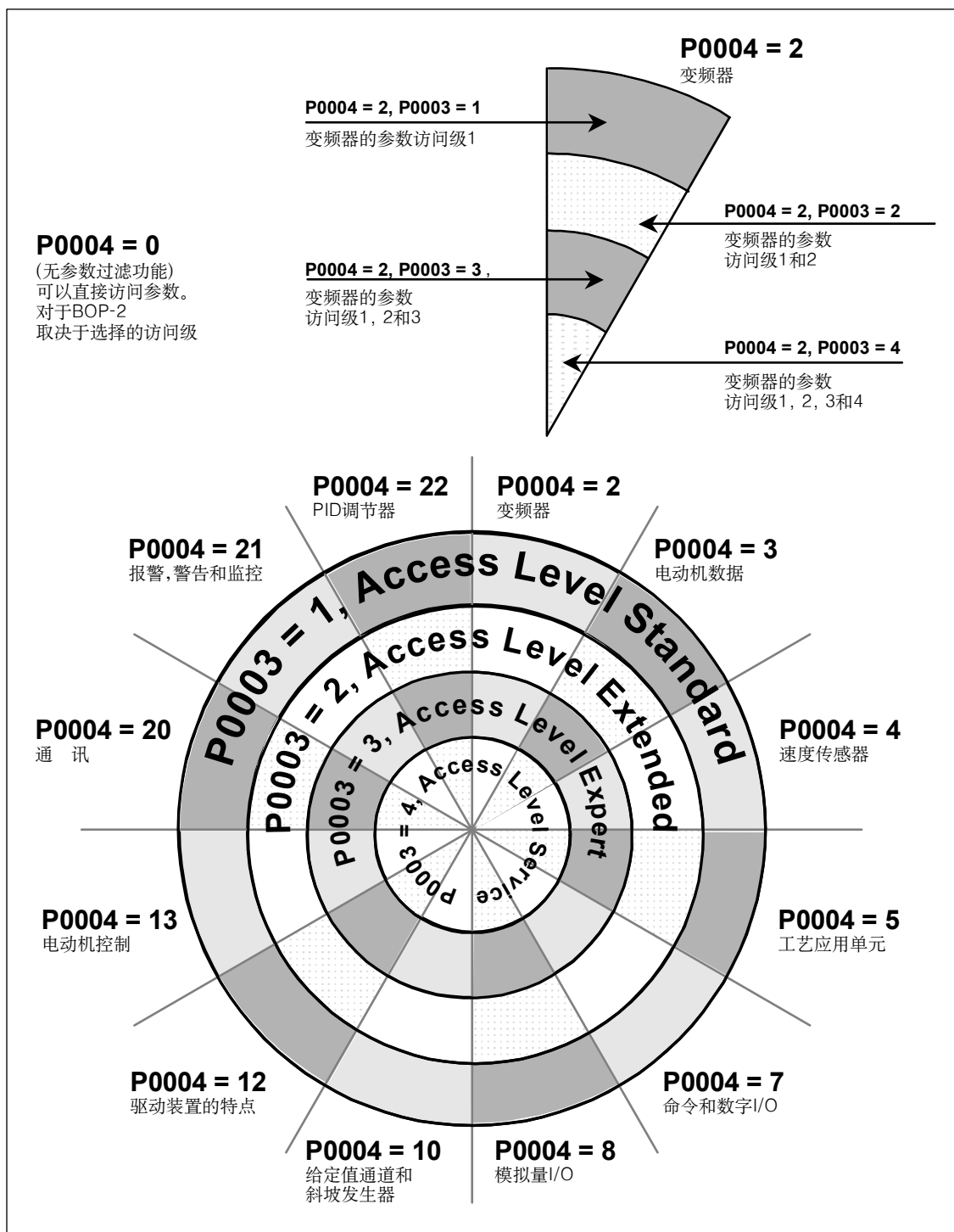
图 5-1 参数概览
