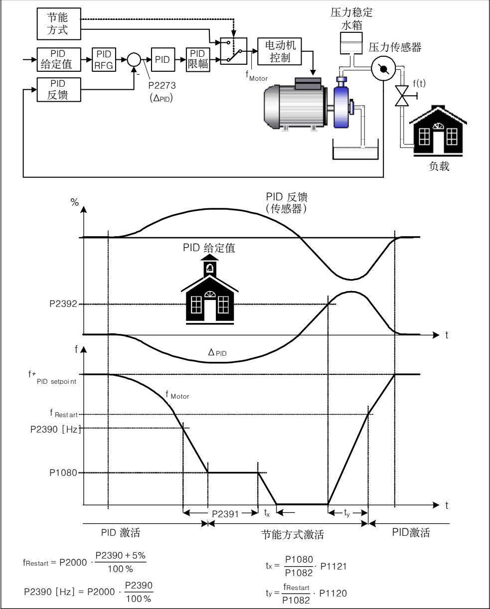
图 4-4 节能方式
