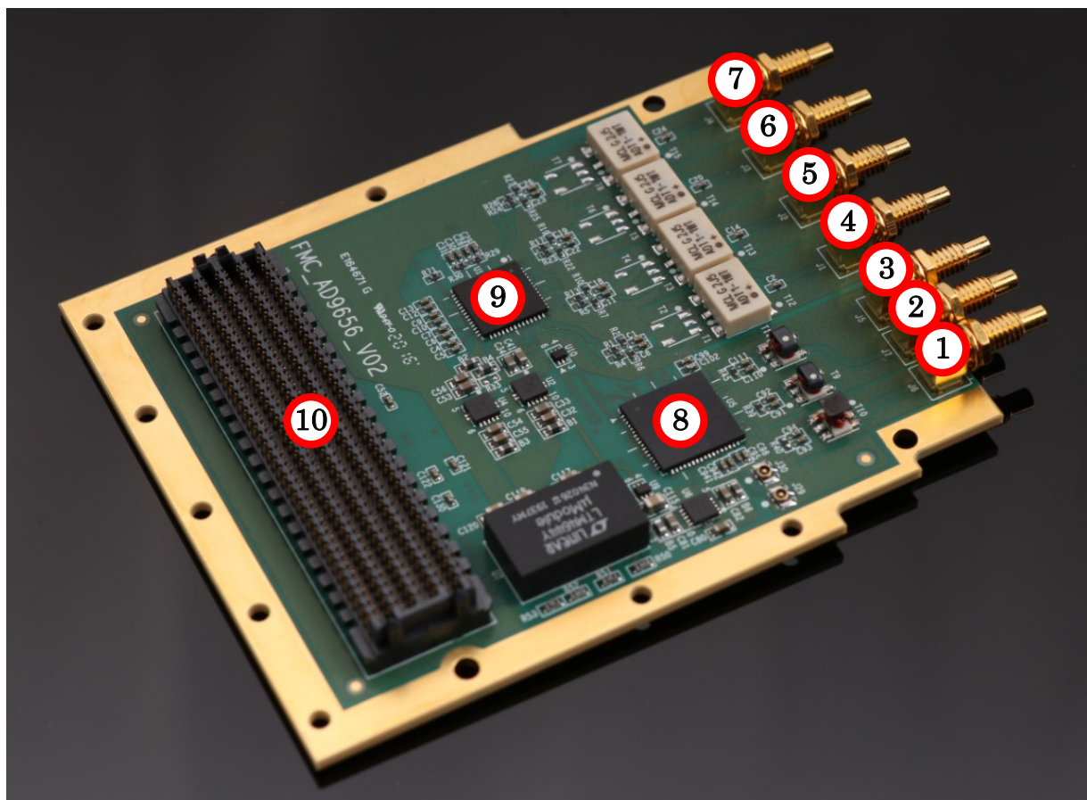
图 2-1 板卡实物图
