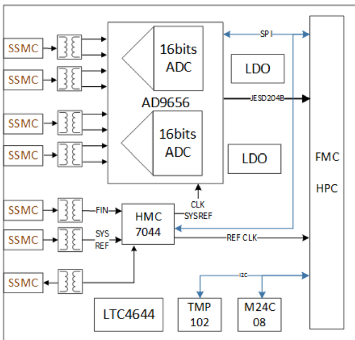
图 1-1 系统结构图
