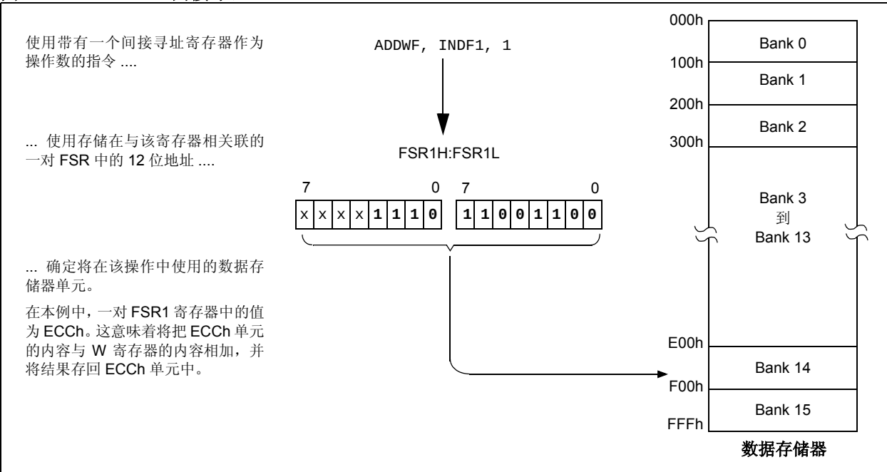
图 5-7：间接寻址
