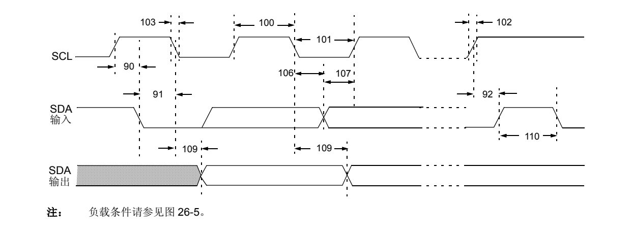
图 26-18: I 2 C™ 总线数据时序
