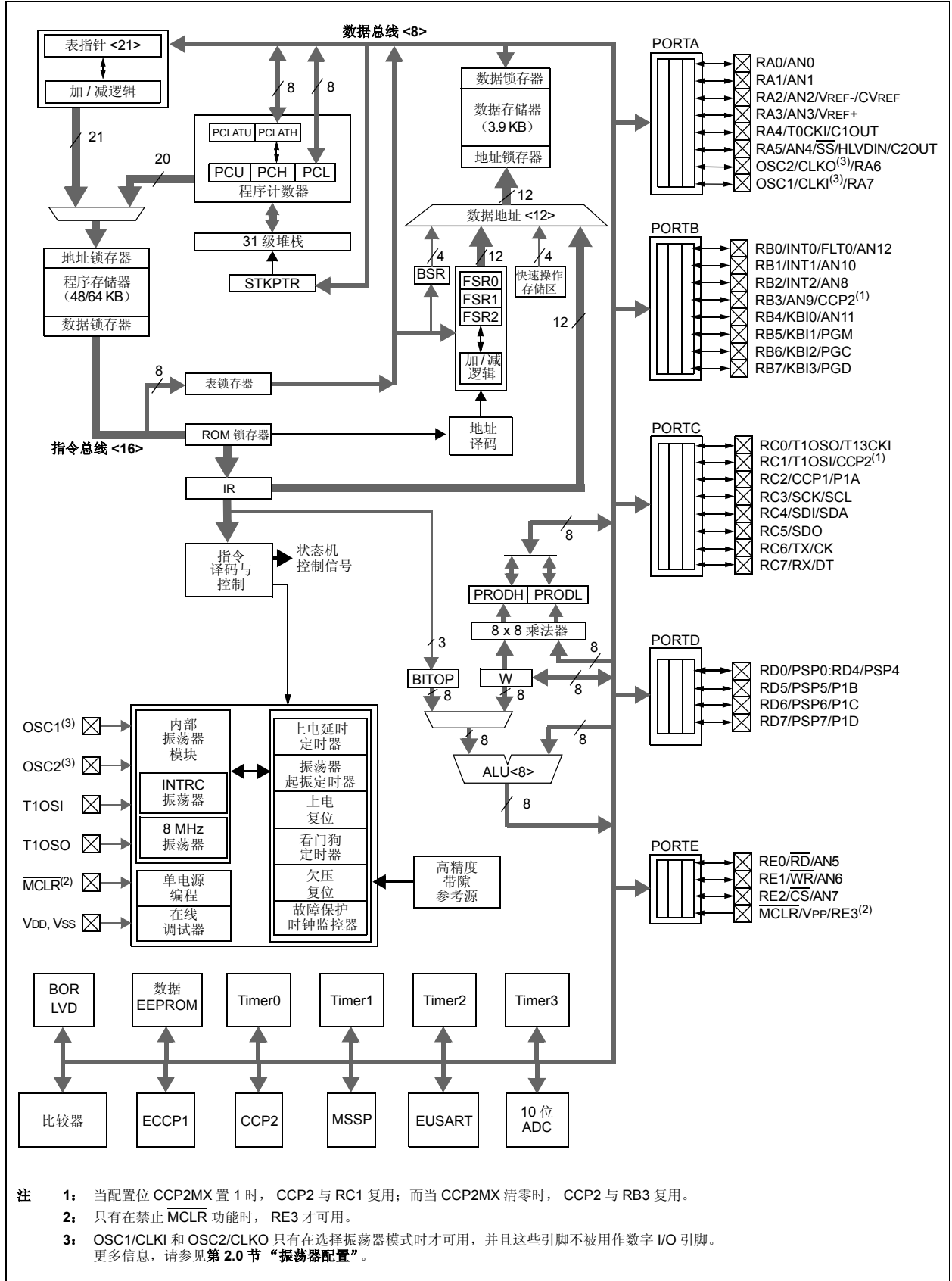
图 1-2: PIC18F4525/4620 (40/44 引脚) 框图
