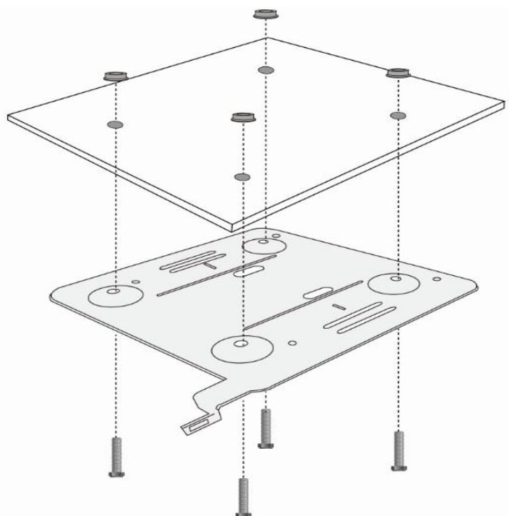
图 3-8 吸顶支架安装示意图
