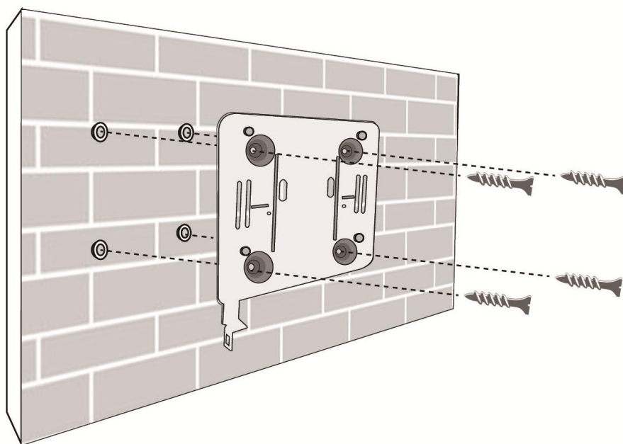
图 3-5 壁挂支架安装示意图
