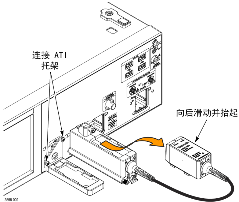
图 6: 安装 ATI 支架并从探头载体上拆下传送梭
