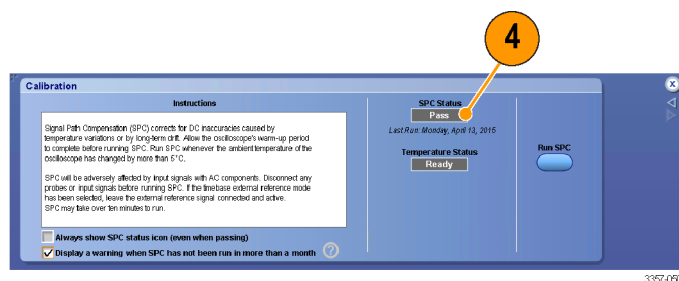
图 20: DPO70000 示波器上的 Calibration（校准）菜单
