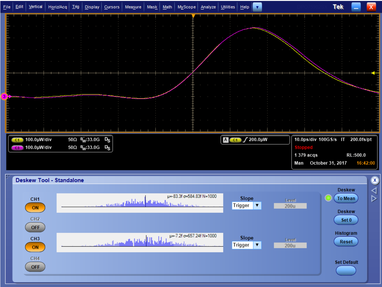
图 15: 最终相差校正过波形的示例
