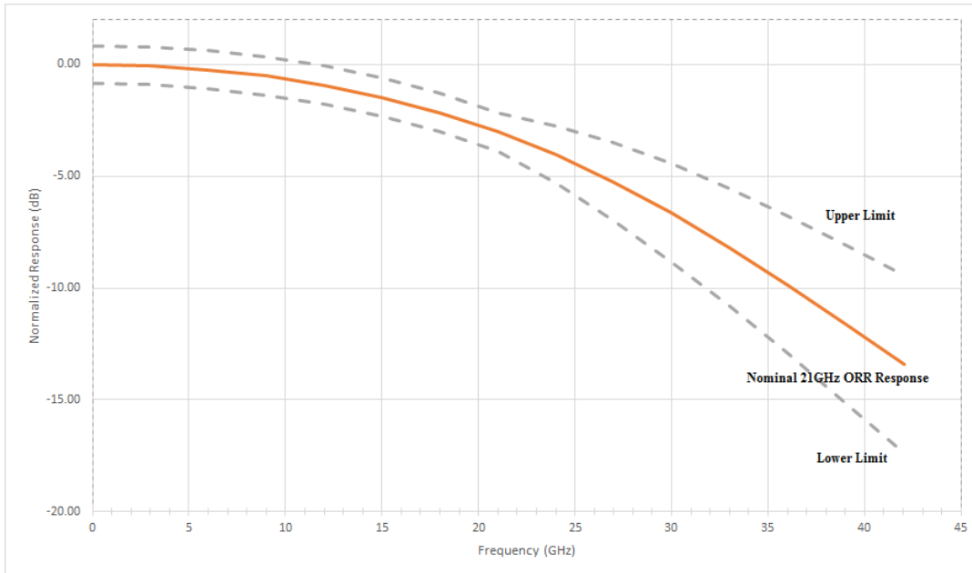
图 22: DPO70E1 光探头和 DPO70000SX ATI 通道的四阶 Bessel-Thompson 频响
