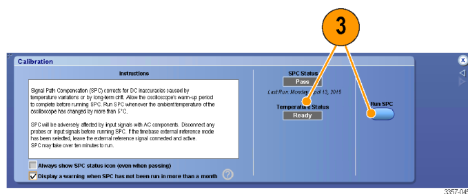
图 19: DPO70000 示波器上的 Calibration（校准）菜单
