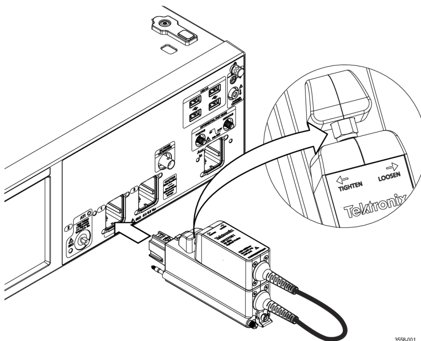
图 5: 将 DPO70E 系列探头连接到示波器
