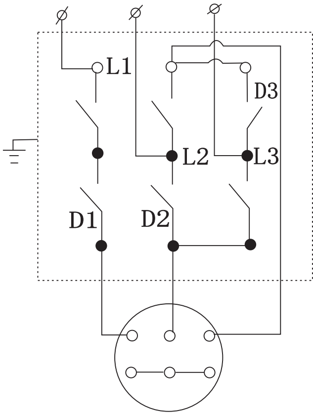
可逆转换开关线路图
