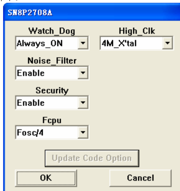
图 2-49 激活状态下的设置对话框
