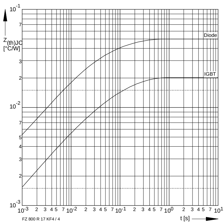
Bild / Fig. 4 Transient innerer Wärmewiderstand (DC) / Transient thermal impedance (DC)
